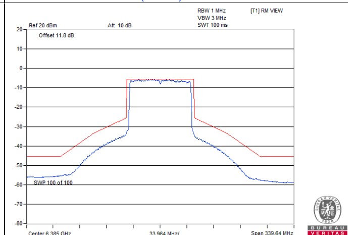
802.11ax (HE80) / Chain 3 : CH 87
