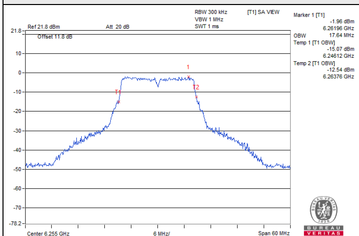
802.11a / Chain 2 : CH 61
