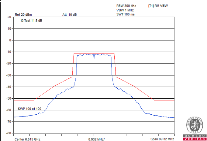
802.11ax (HE20) / Chain 2 : CH 113
