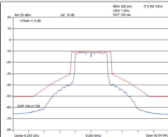
802.11ax (HE20) / Chain 0 : CH 61
