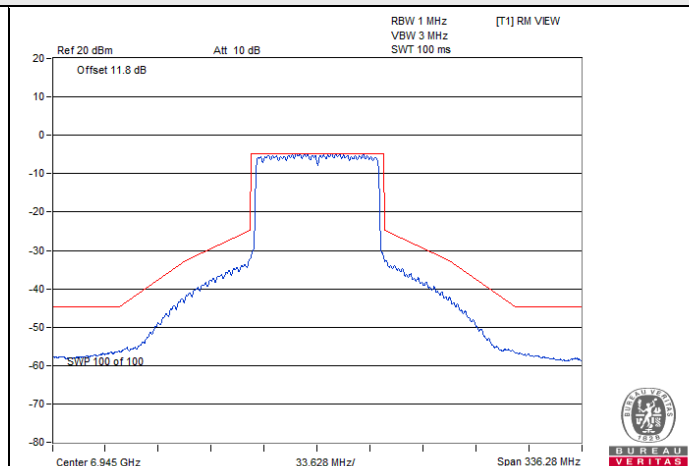
802.11ax (HE80) / Chain 2 : CH 199
