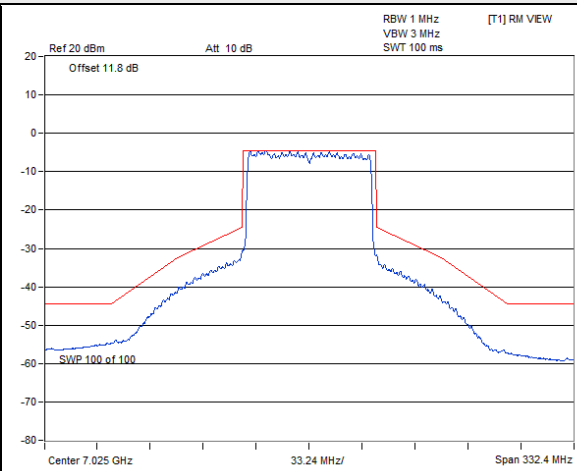
802.11ax (HE80) / Chain 3 : CH 215
