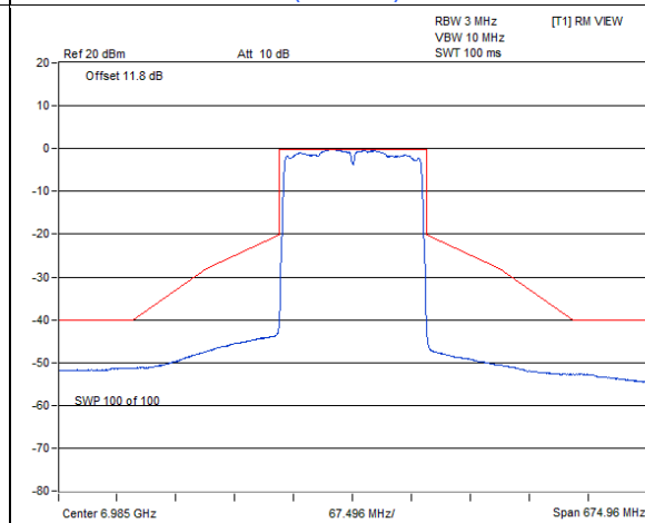
802.11ax (HE160) / Chain 0 : CH 207
