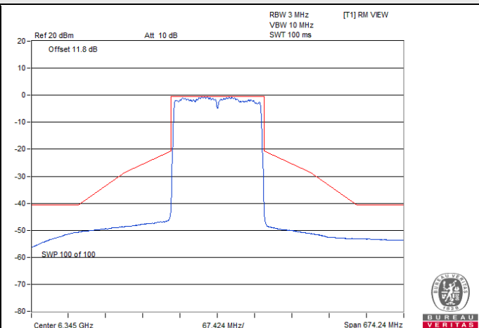
802.11ax (HE160) / Chain 1 : CH 79
