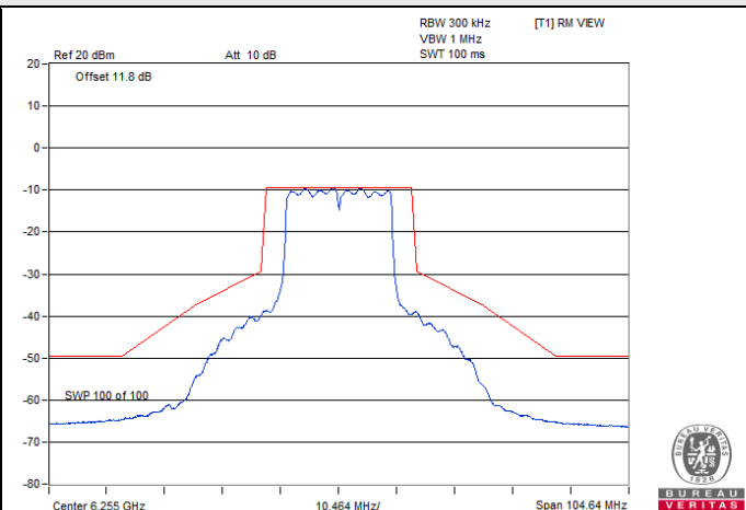
802.11ax (HE20) / Chain 2 : CH 61
