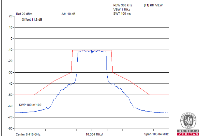
802.11ax (HE20) / Chain 2 : CH 93
