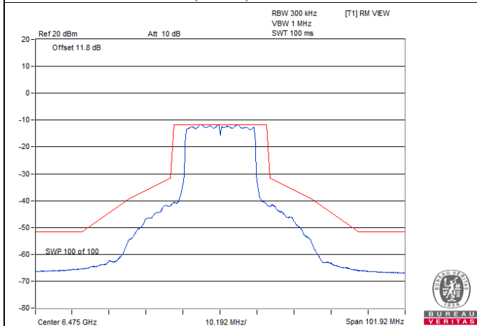
802.11ax (HE20) / Chain 2 : CH 105
