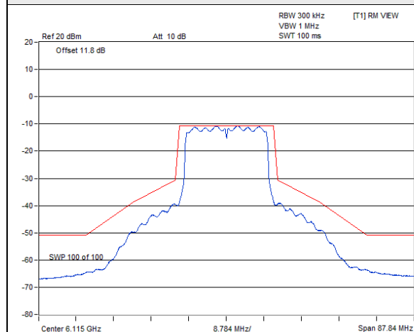
802.11ax (HE20) / Chain 0 : CH 33
