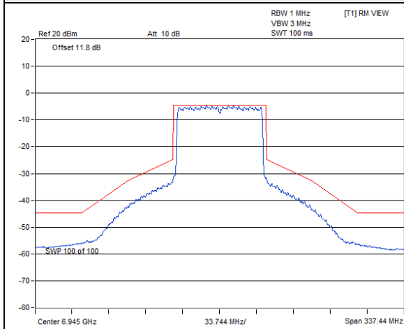
802.11ax (HE80) / Chain 3 : CH 199
