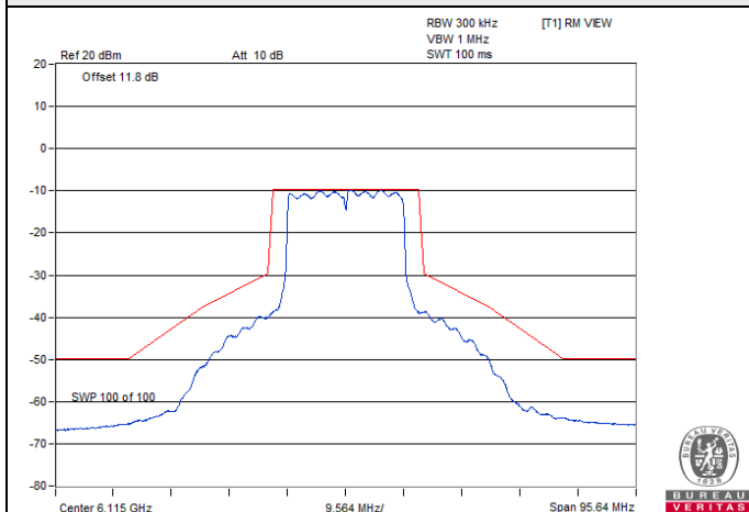
802.11ax (HE20) / Chain 2 : CH 33
