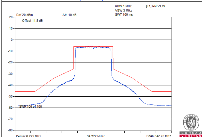
802.11ax (HE80) / Chain 3 : CH 55
