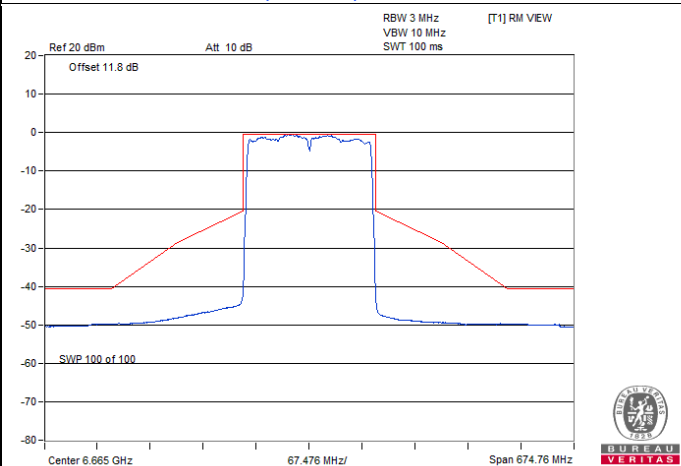
802.11ax (HE160) / Chain 1 : CH 143
