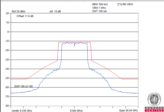
802.11ax (HE20) / Chain 2 : CH 97
