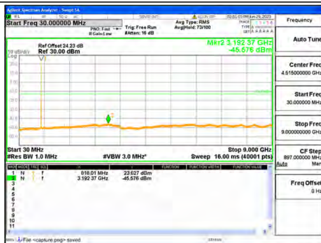
26 Part90 / 3MHz / Mid CH / QPSK
