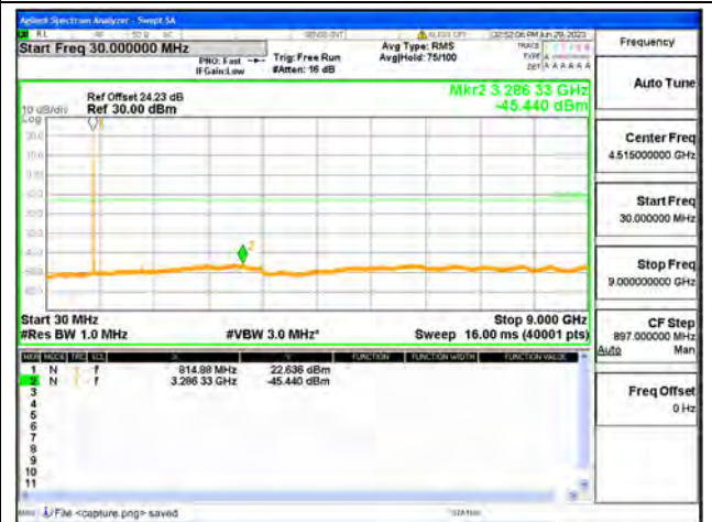
26 Part90 / 10MHz / Mid CH / QPSK
