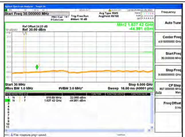
26 Part90 / 1.4MHz / Mid CH / QPSK
