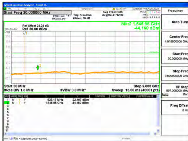
26 Part90 / 1.4MHz / High CH / QPSK
