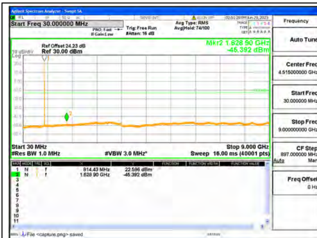
26 Part90 / 5MHz / Low CH / QPSK
