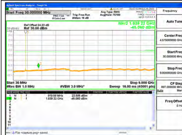
26 Part90 / 5MHz / High CH / QPSK
