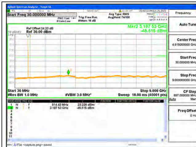
26 Part90 / 1.4MHz / Low CH / QPSK
