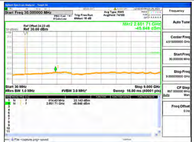
26 Part90 / 3MHz / Low CH / QPSK
