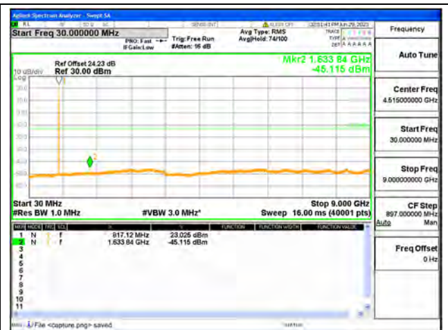
26 Part90 / 5MHz / Mid CH / QPSK
