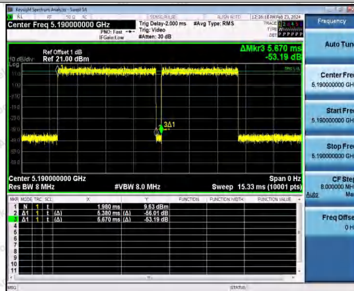
11AX40MIMO_Ant2_5190
