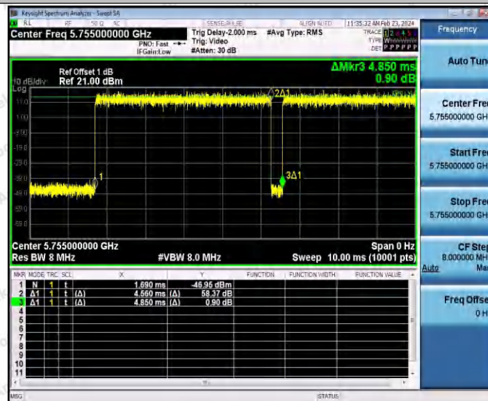
11AC40MIMO_Ant2_5755
