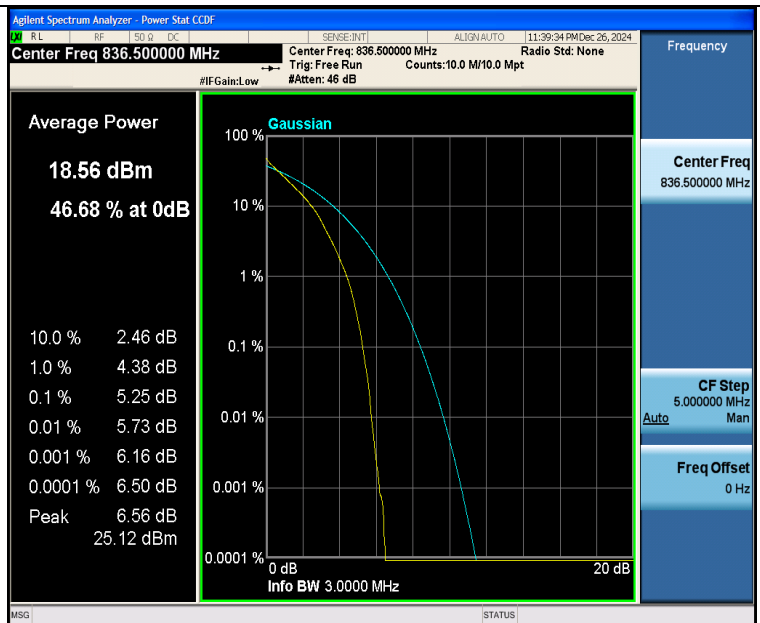
Band26(824-849)-3MHz-QPSK-26915-15RB#0-PASS
