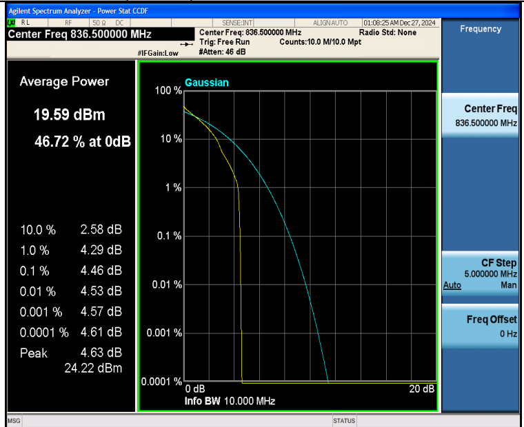
Band26(824-849)-10MHz-QPSK-26915-1RB#0-PASS
