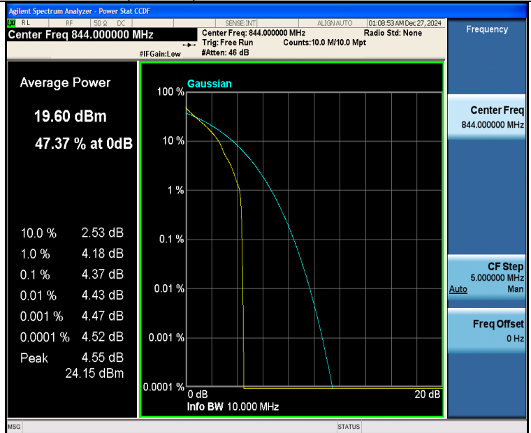
Band26(824-849)-10MHz-QPSK-26990-1RB#0-PASS
