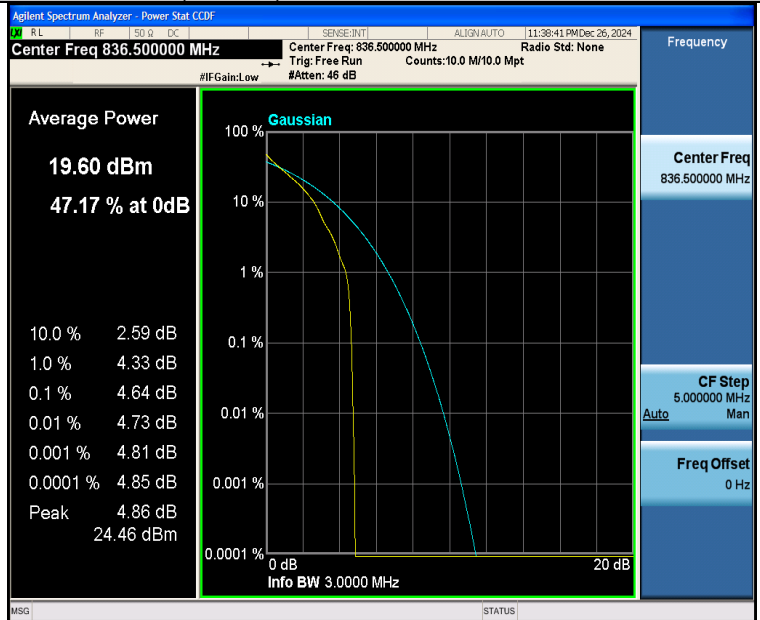
Band26(824-849)-3MHz-QPSK-26915-1RB#0-PASS
