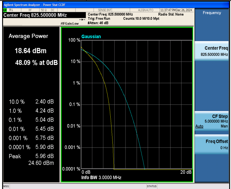
Band26(824-849)-3MHz-QPSK-26805-15RB#0-PASS
