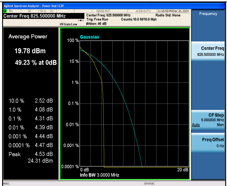
Band26(824-849)-3MHz-QPSK-26805-1RB#0-PASS
