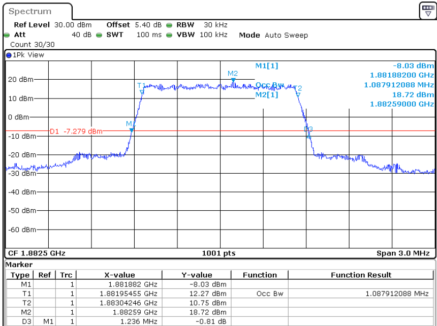
Band25-1.4MHz-QPSK-26365-6RB#0-1.088
