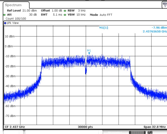
11N20SISO_Ant1_2437
