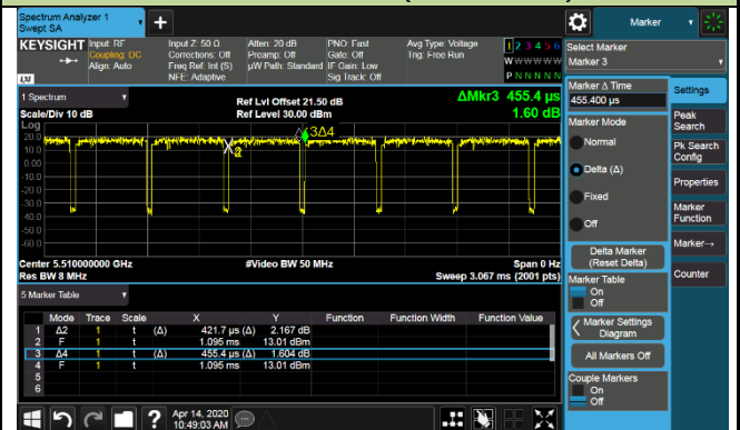
802.11ax-HE40 (T=421.7us)
