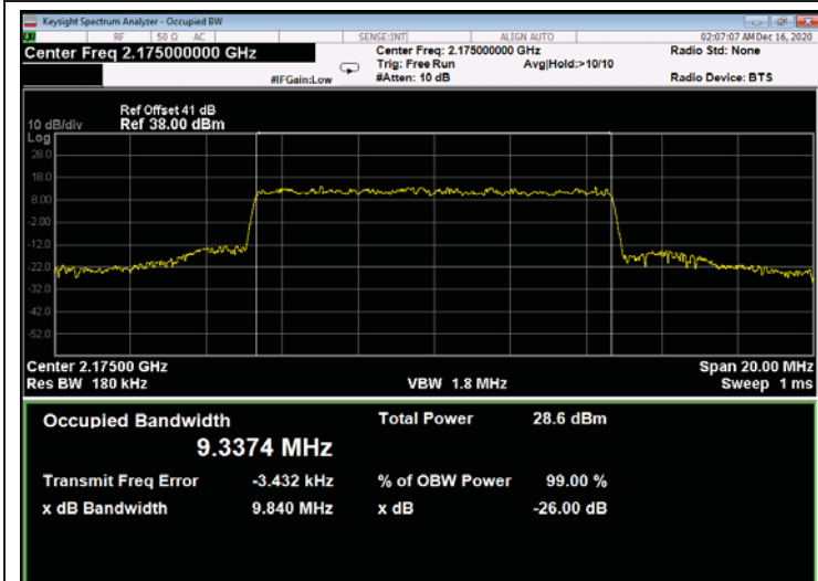
Figure 747: QPSK 10MHz B.W.; 2175.0MHz, 15kHz - Output
