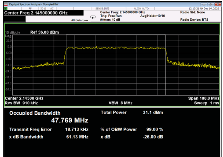
Figure 790: QPSK 50MHz B.W.; 2145.0MHz, 30kHz - Output
