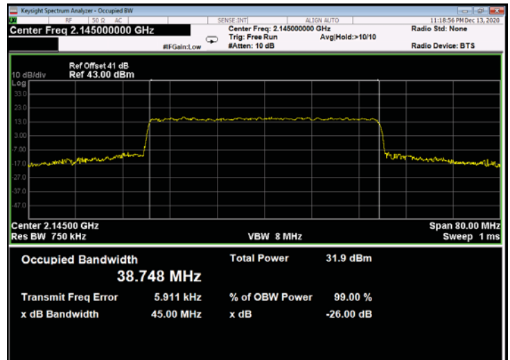
Figure 780: QPSK 40MHz B.W.; 2145.0MHz, 15kHz - Output
