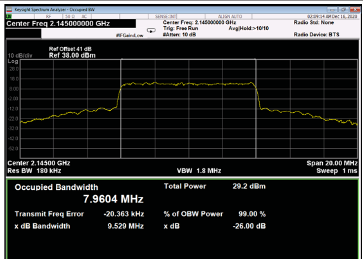
Figure 746: QPSK 10MHz B.W.; 2145.0MHz, 60kHz - Output
