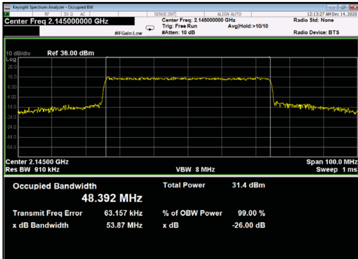
Figure 789: QPSK 50MHz B.W.; 2145.0MHz, 15kHz - Output
