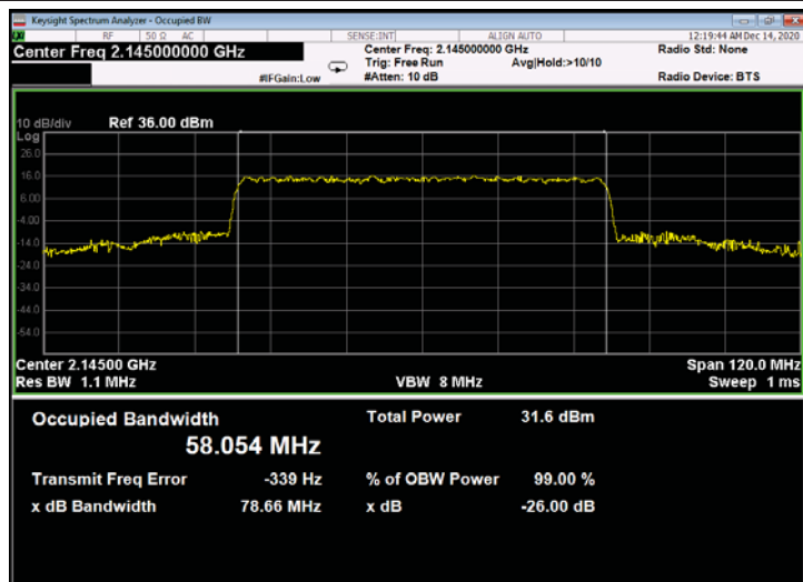
Figure 797: QPSK 60MHz B.W.; 2145.0MHz, 30kHz - Output
