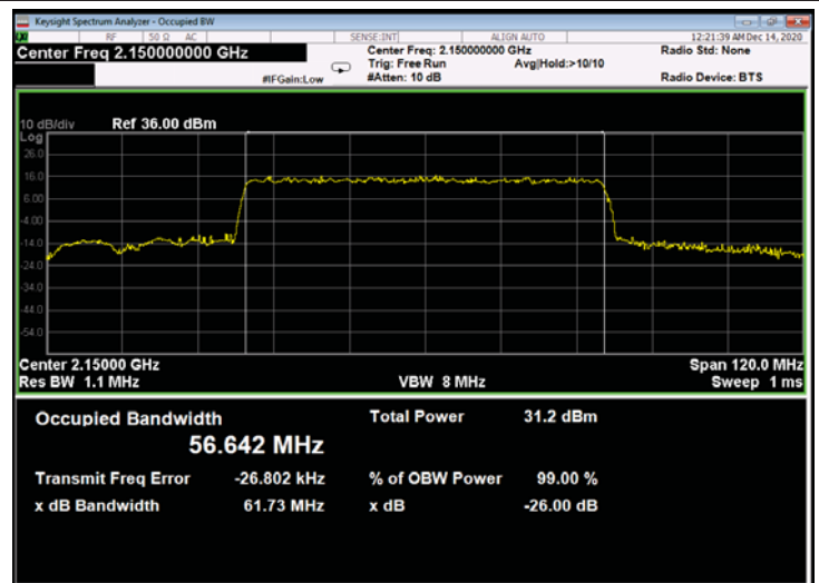
Figure 800: QPSK 60MHz B.W.; 2150.0MHz, 60kHz - Output
