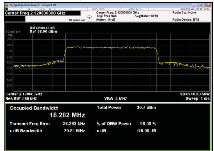
Figure 760: QPSK 20MHz B.W.; 2120.0MHz, 30kHz - Output
