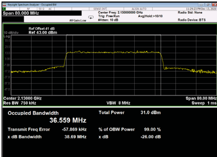
Figure 779: QPSK 40MHz B.W.; 2130.0MHz, 60kHz - Output
