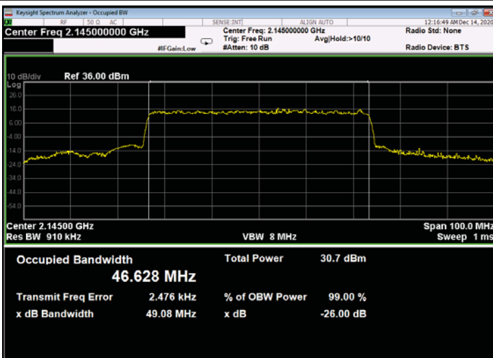
Figure 791: QPSK 50MHz B.W.; 2145.0MHz, 60kHz - Output
