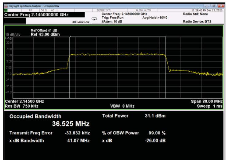
Figure 782: QPSK 40MHz B.W.; 2145.0MHz, 60kHz - Output
