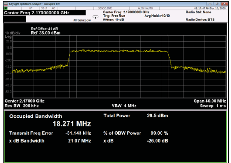
Figure 766: QPSK 20MHz B.W.; 2170.0MHz, 30kHz - Output
