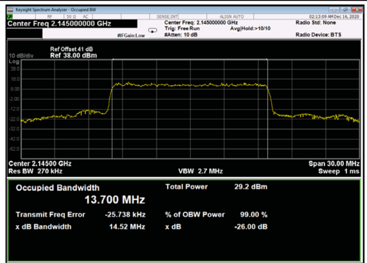
Figure 754: QPSK 15MHz B.W.; 2145.0MHz, 30kHz - Output
