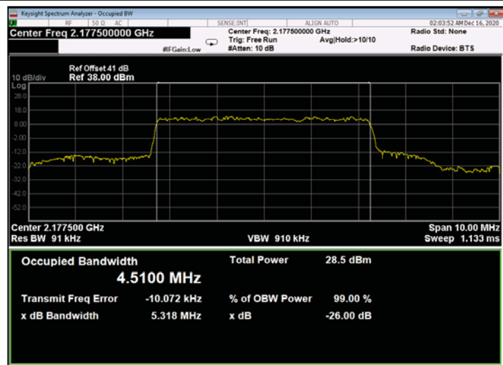
Figure 739: QPSK 5MHz B.W.; 2177.5MHz, 15kHz - Output
