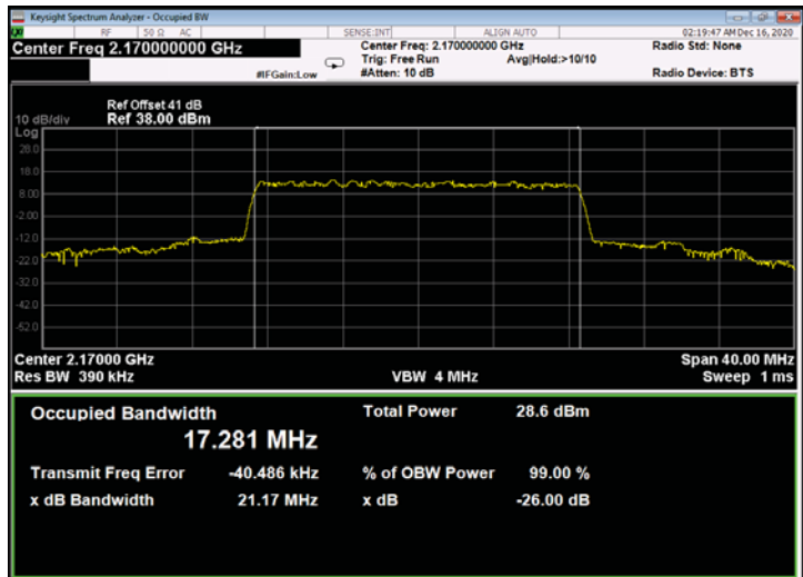
Figure 767: QPSK 20MHz B.W.; 2170.0MHz, 60kHz - Output
