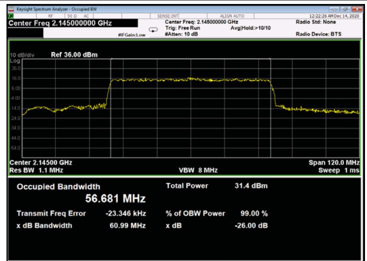
Figure 798: QPSK 60MHz B.W.; 2145.0MHz, 60kHz - Output
