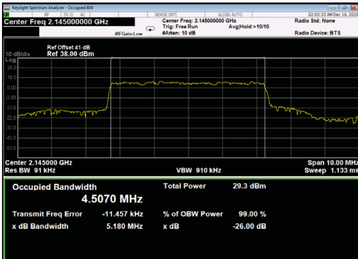
Figure 737: QPSK 5MHz B.W.; 2145.0MHz, 15kHz - Output
