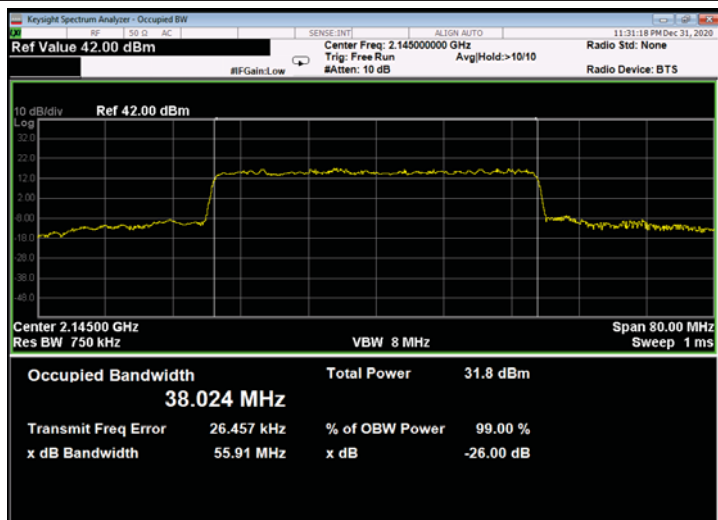
Figure 781: QPSK 40MHz B.W.; 2145.0MHz, 30kHz - Output
