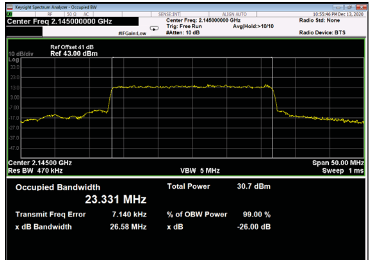
Figure 772: QPSK 25MHz B.W.; 2145.0MHz, 30kHz - Output
