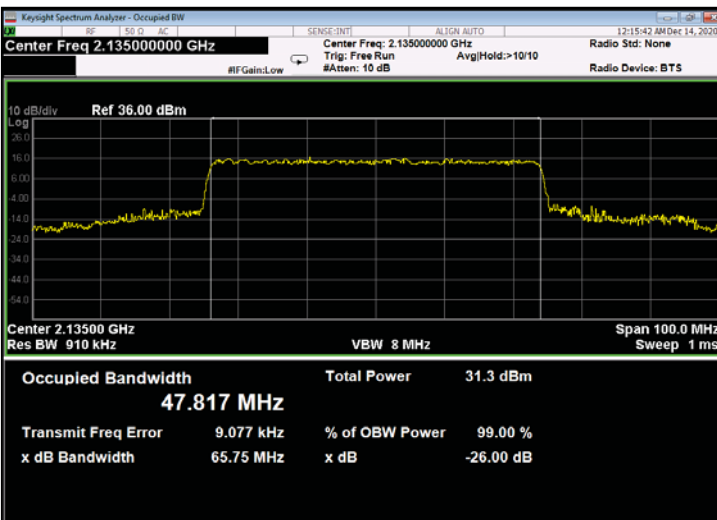
Figure 787: QPSK 50MHz B.W.; 2135.0MHz, 30kHz - Output
