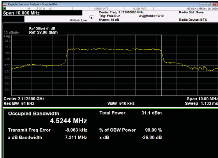
Figure 735: QPSK 5MHz B.W.; 2112.5MHz, 15kHz - Output
