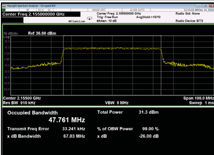
Figure 793: QPSK 50MHz B.W.; 2155.0MHz, 30kHz - Output
