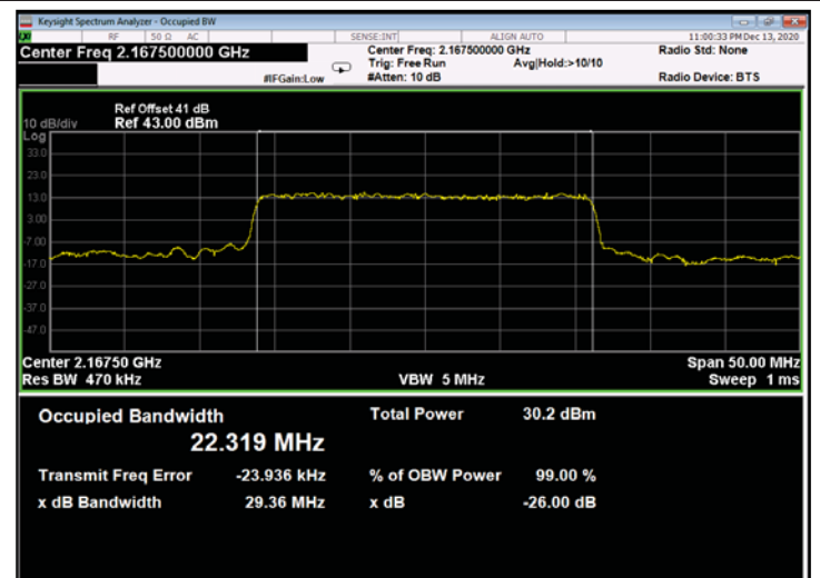
Figure 776: QPSK 25MHz B.W.; 2167.5MHz, 60kHz - Output
