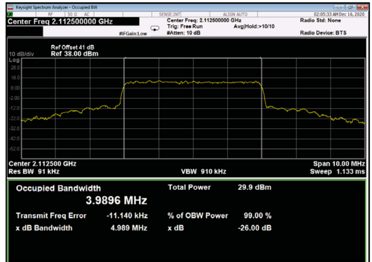
Figure 736: QPSK 5MHz B.W.; 2112.5MHz, 30kHz - Output
