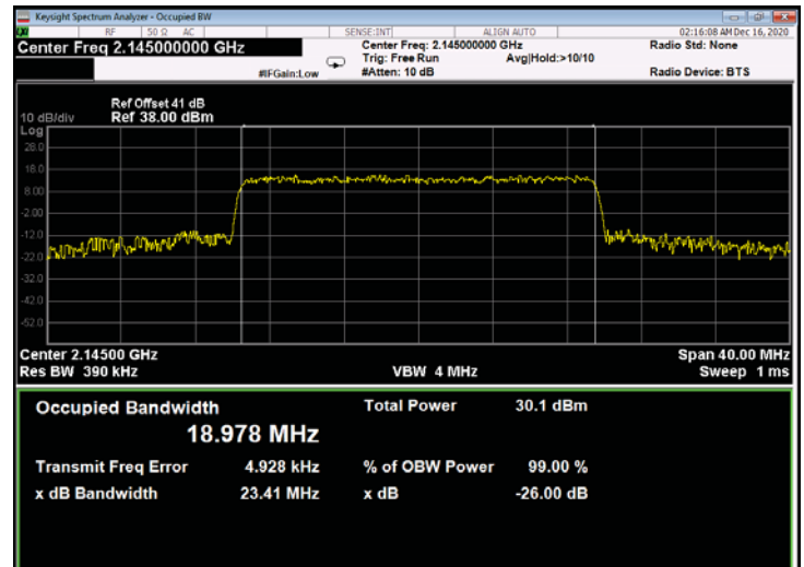
Figure 762: QPSK 20MHz B.W.; 2145.0MHz, 15kHz - Output
