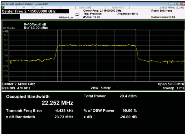
Figure 773: QPSK 25MHz B.W.; 2145.0MHz, 60kHz - Output
