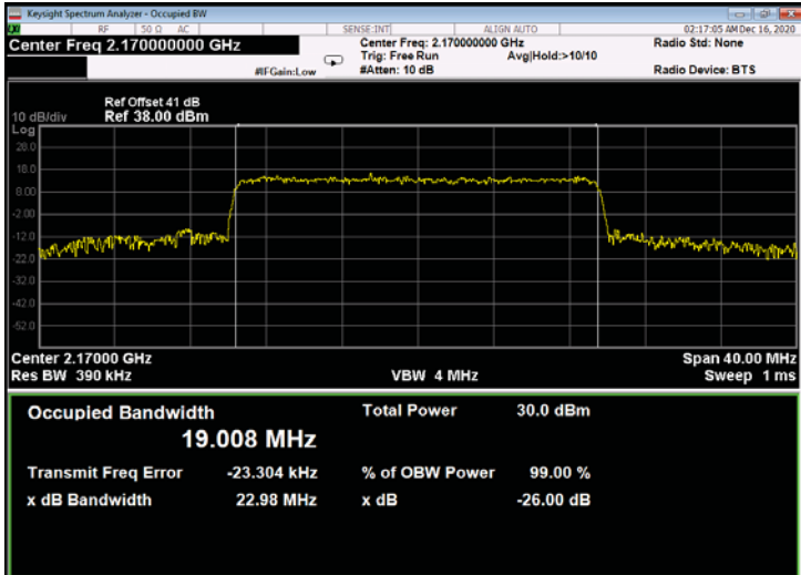
Figure 765: QPSK 20MHz B.W.; 2170.0MHz, 15kHz - Output
