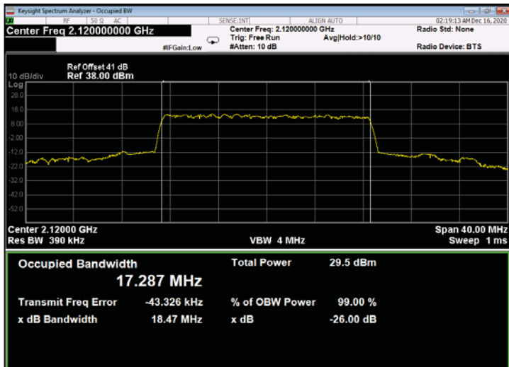
Figure 761: QPSK 20MHz B.W.; 2120.0MHz, 60kHz - Output
