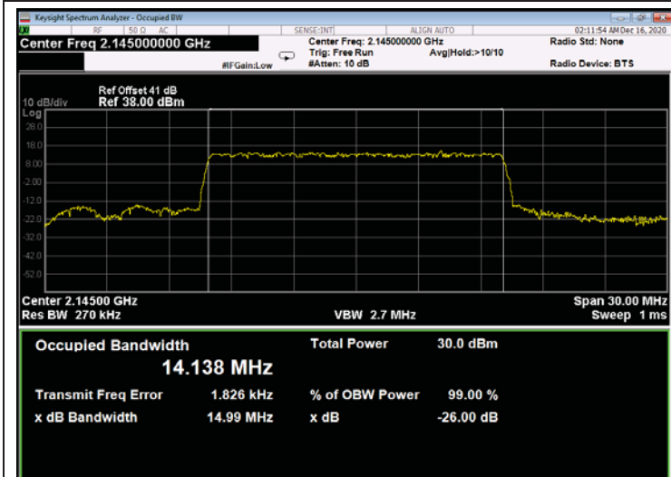
Figure 753: QPSK 15MHz B.W.; 2145.0MHz, 15kHz - Output
