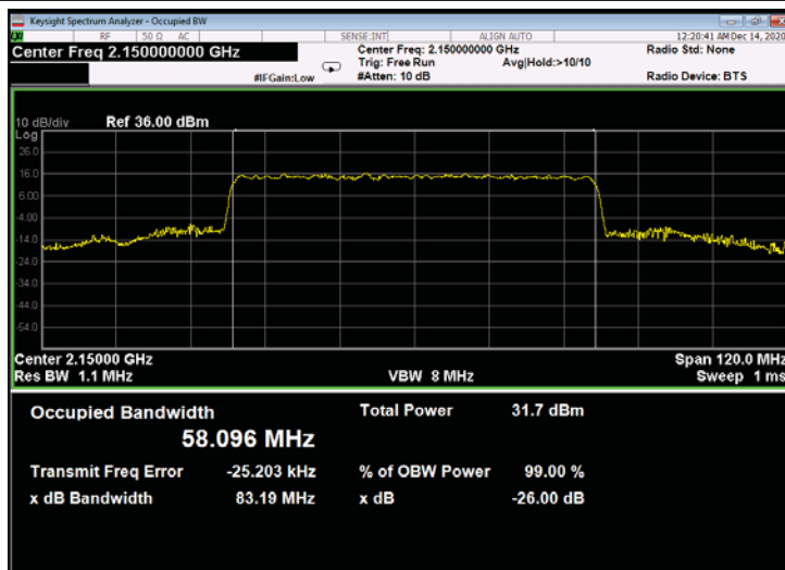
Figure 799: QPSK 60MHz B.W.; 2150.0MHz, 30kHz - Output
