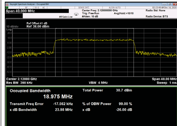
Figure 759: QPSK 20MHz B.W.; 2120.0MHz, 15kHz - Output
