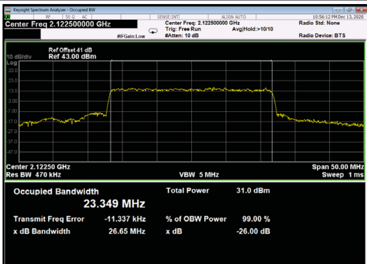
Figure 769: QPSK 25MHz B.W.; 2122.5MHz, 30kHz - Output
