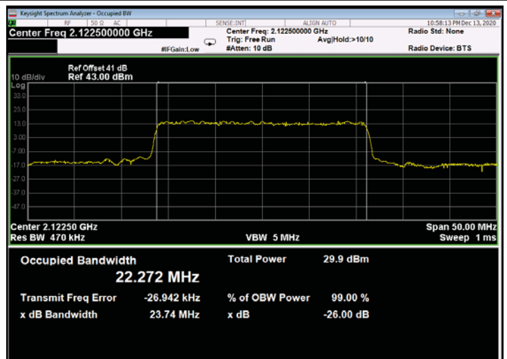
Figure 770: QPSK 25MHz B.W.; 2122.5MHz, 60kHz - Output
