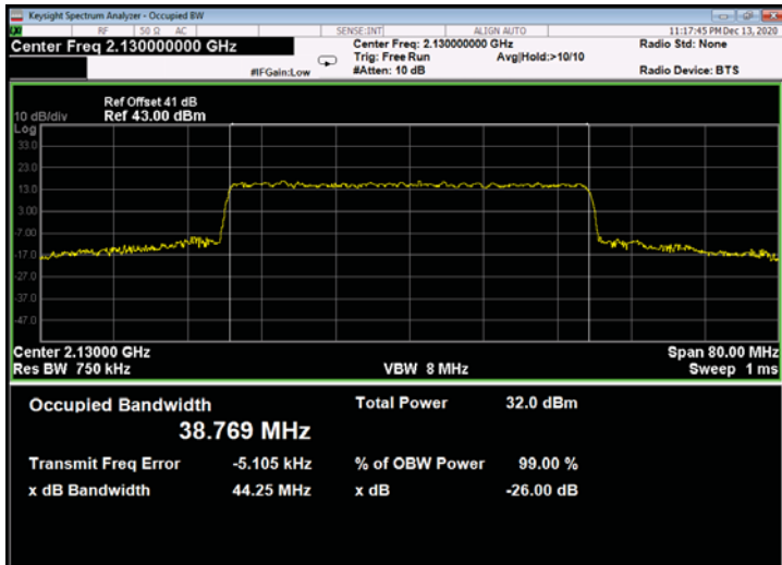
Figure 777: QPSK 40MHz B.W.; 2130.0MHz, 15kHz - Output
