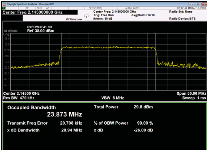
Figure 771: QPSK 25MHz B.W.; 2145.0MHz, 15kHz - Output
