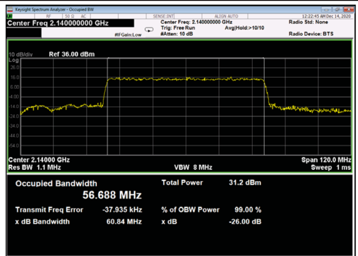
Figure 796: QPSK 60MHz B.W.; 2140.0MHz, 60kHz - Output
