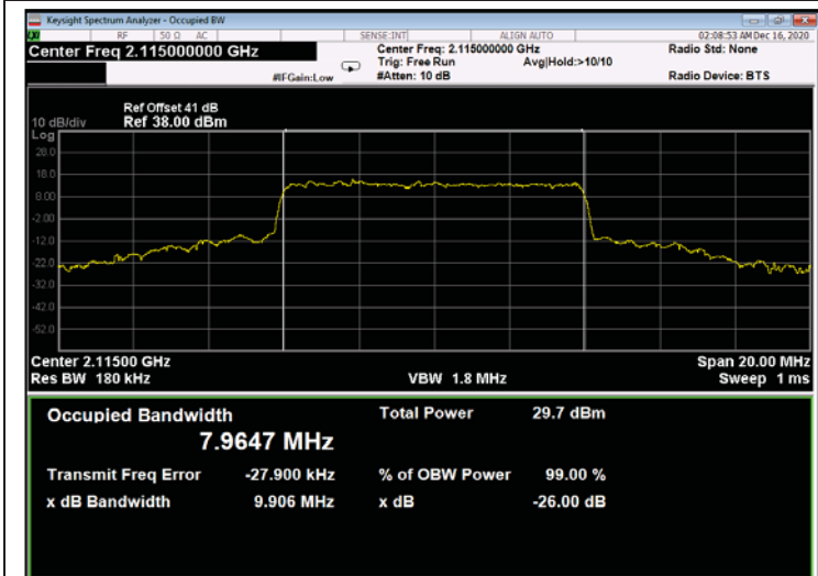
Figure 743: QPSK 10MHz B.W.; 2115.0MHz, 60kHz - Output
