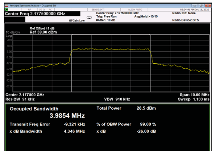
Figure 740: QPSK 5MHz C.S.; 2177.5MHz, 30kHz - Output
