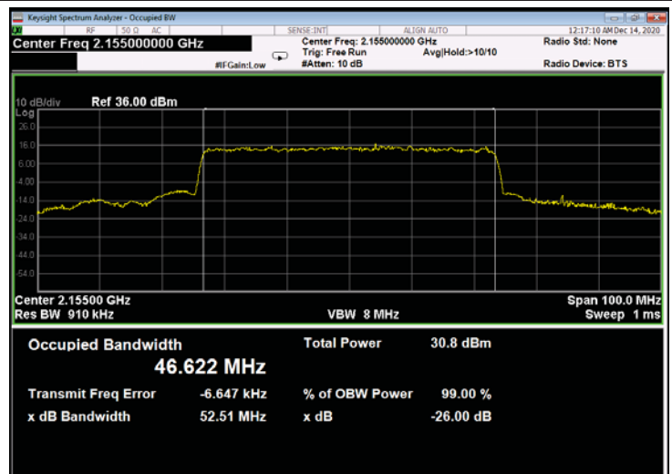
Figure 794: QPSK 50MHz B.W.; 2155.0MHz, 60kHz - Output
