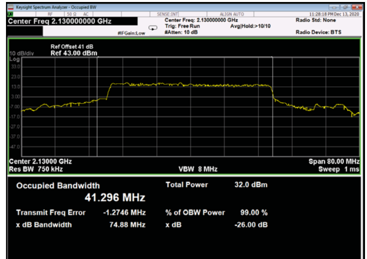
Figure 778: QPSK 40MHz B.W.; 2130.0MHz, 30kHz - Output
