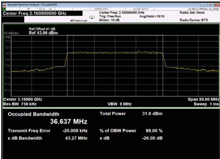
Figure 785: QPSK 40MHz B.W.; 2160.0MHz, 60kHz - Output
