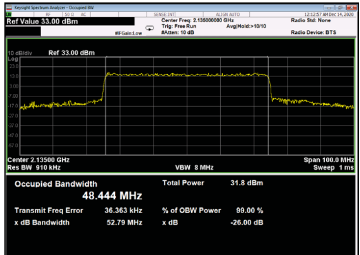
Figure 786: QPSK 50MHz B.W.; 2135.0MHz, 15kHz - Output
