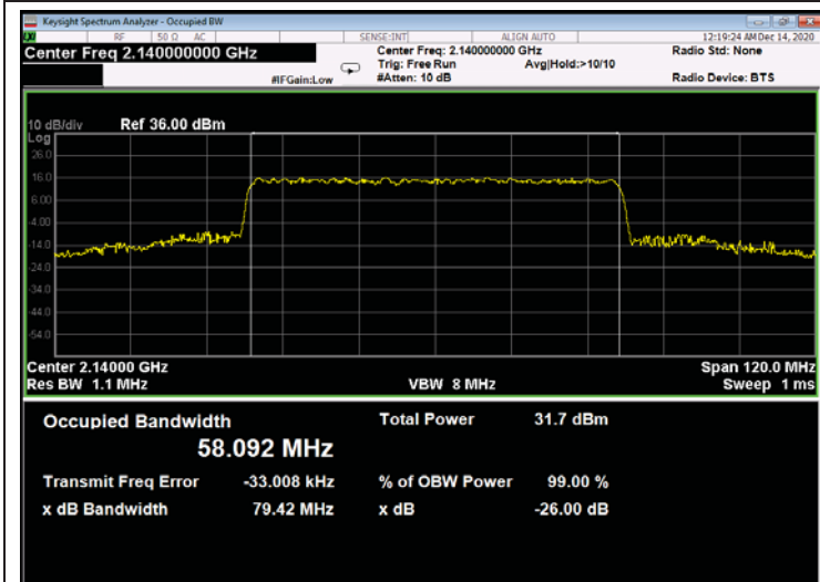
Figure 795: QPSK 60MHz B.W.; 2140.0MHz, 30kHz - Output
