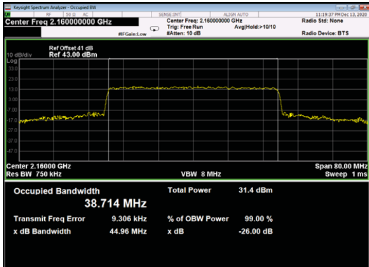
Figure 783: QPSK 40MHz B.W.; 2160.0MHz, 15kHz - Output
