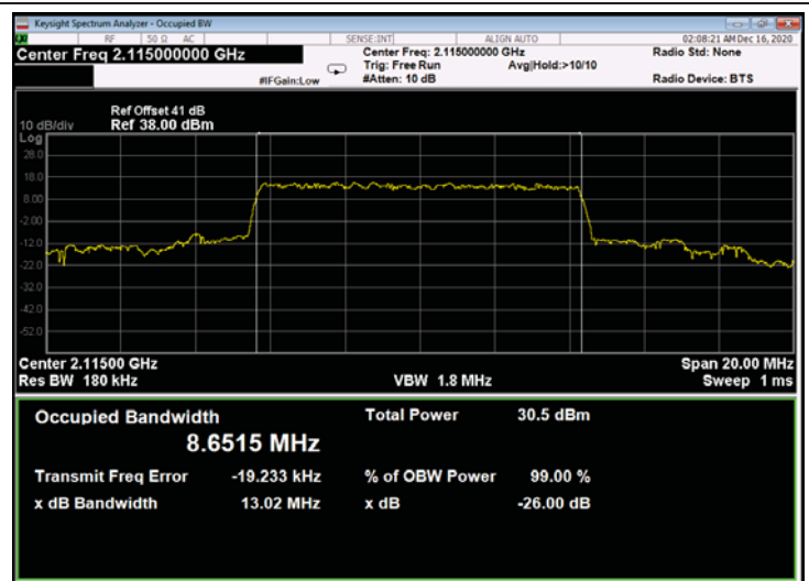
Figure 742: QPSK 10MHz B.W.; 2115.0MHz, 30kHz - Output
