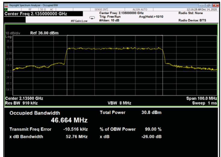
Figure 788: QPSK 50MHz B.W.; 2135.0MHz, 60kHz - Output
