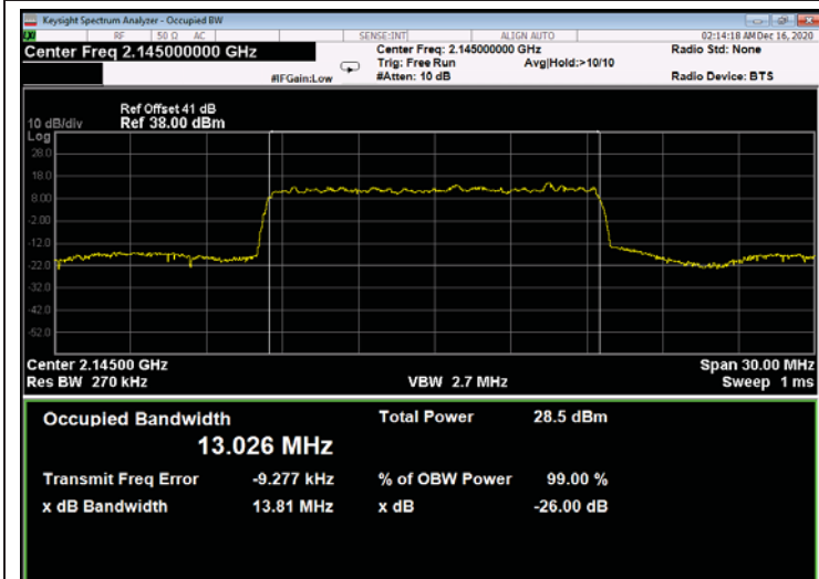
Figure 755: QPSK 15MHz B.W.; 2145.0MHz, 60kHz - Output
