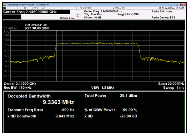
Figure 744: QPSK 10MHz B.W.; 2145.0MHz, 15kHz - Output
