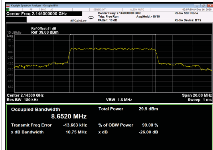
Figure 745: QPSK 10MHz B.W.; 2145.0MHz, 30kHz - Output
