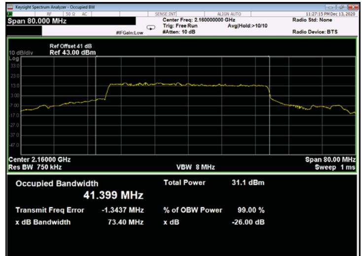
Figure 784: QPSK 40MHz B.W.; 2160.0MHz, 30kHz - Output
