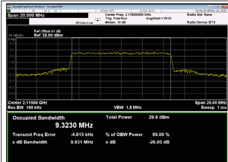
Figure 741: QPSK 10MHz B.W.; 2115.0MHz, 15kHz - Output
