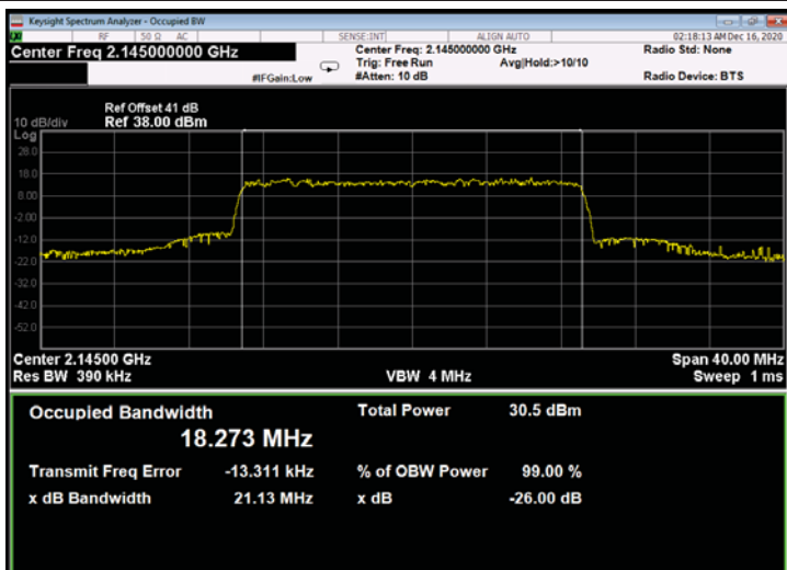
Figure 763: QPSK 20MHz B.W.; 2145.0MHz, 30kHz - Output
