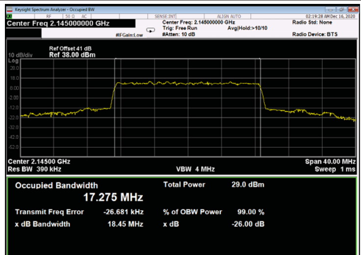
Figure 764: QPSK 20MHz B.W.; 2145.0MHz, 60kHz - Output
