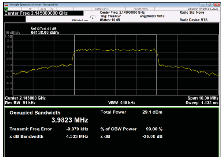
Figure 738: QPSK 5MHz B.W.; 2145.0MHz, 30kHz - Output
