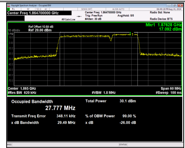
2-2-20MHz-10MHz-QPSK-QPSK-18700-18844-100RB#0- 50RB#0-PASS
