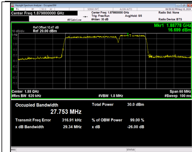
2-2-20MHz-10MHz-QPSK-QPSK-18851-18995-100RB#0-50RB#0-PASS
