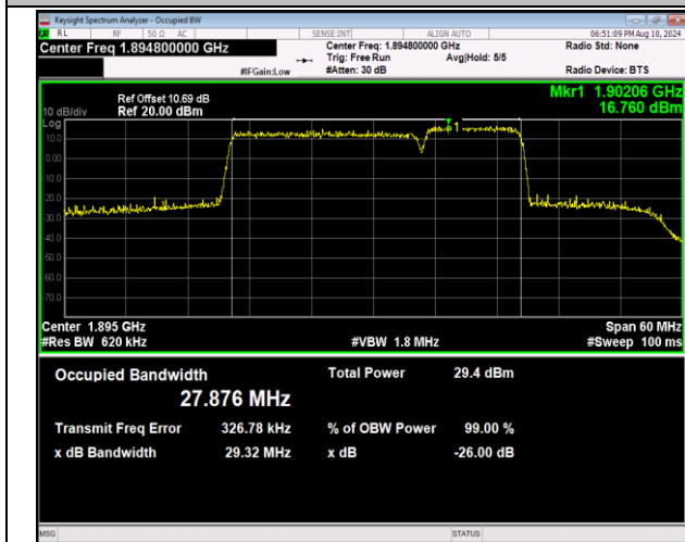
2-2-20MHz-10MHz-16QAM-16QAM-19001-19145-100RB#0-50RB#0-PASS
