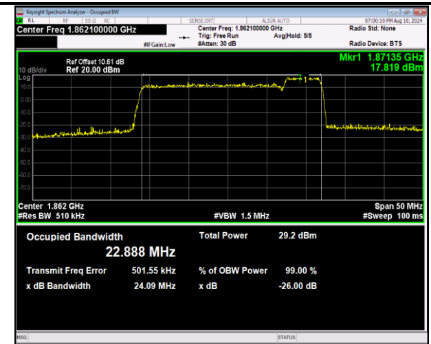
2-2-20MHz-5MHz-16QAM-16QAM-18700-18817-100RB#0 -25RB#0-PASS
