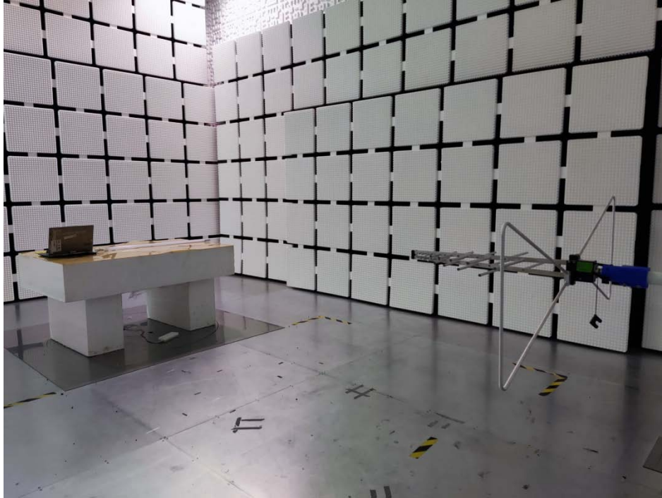
RSE 30MHz-1000MHz
