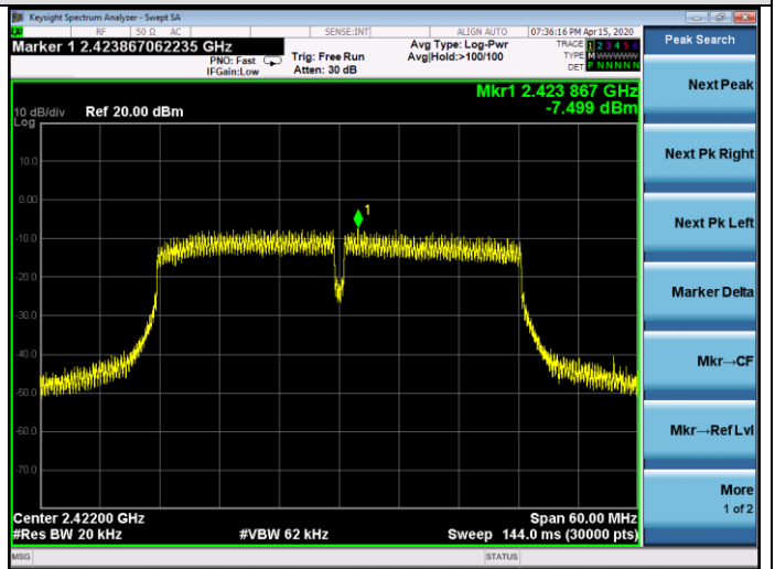
11nHT40-LCH
