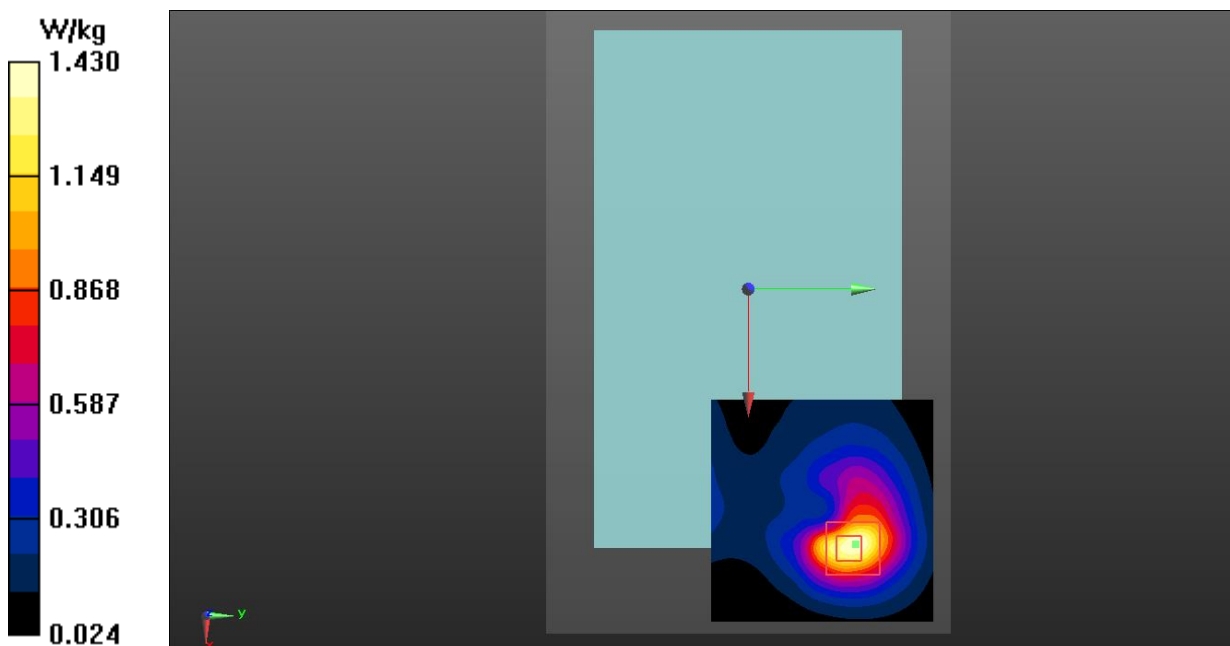
Fig. 2 GSM1900 Body
