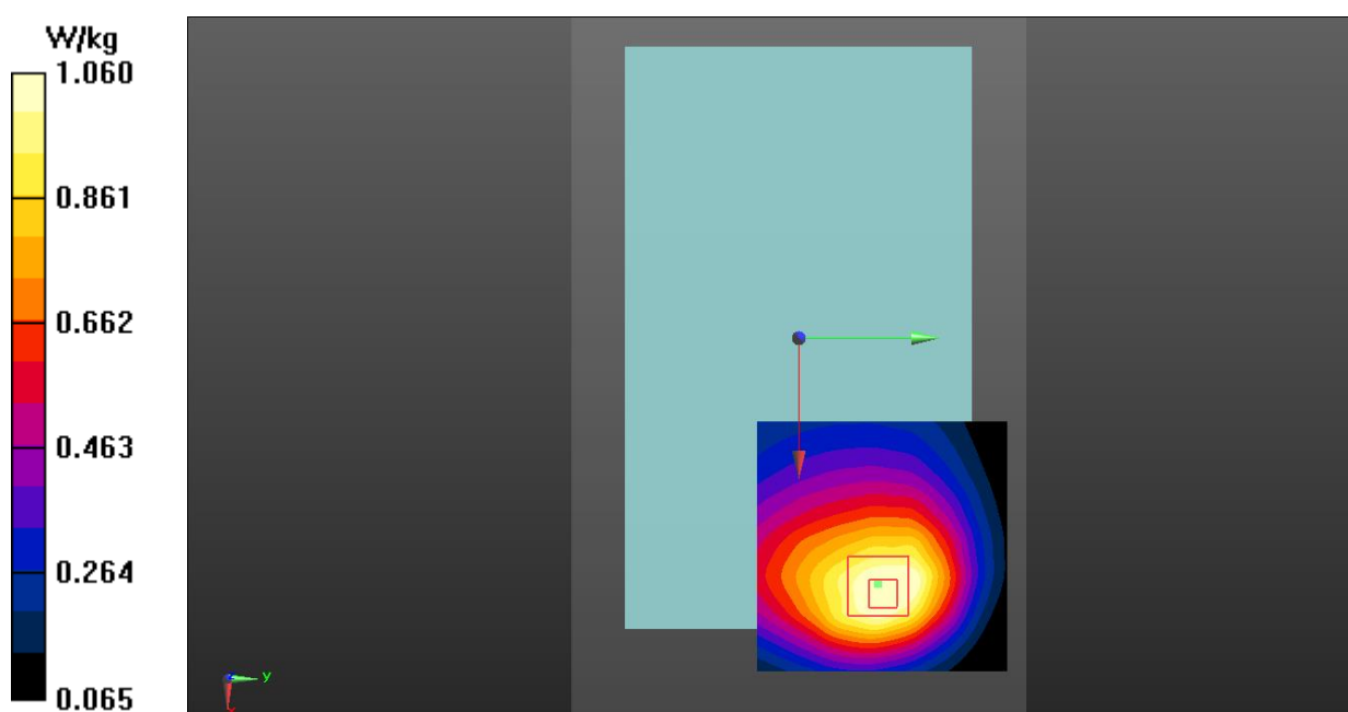
Fig. 1 GSM850 Body
