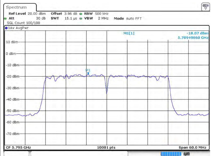
PSD n40 5795MHz Ant2
