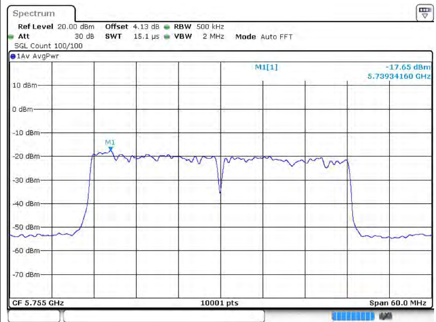
PSD n40 5755MHz Ant2
