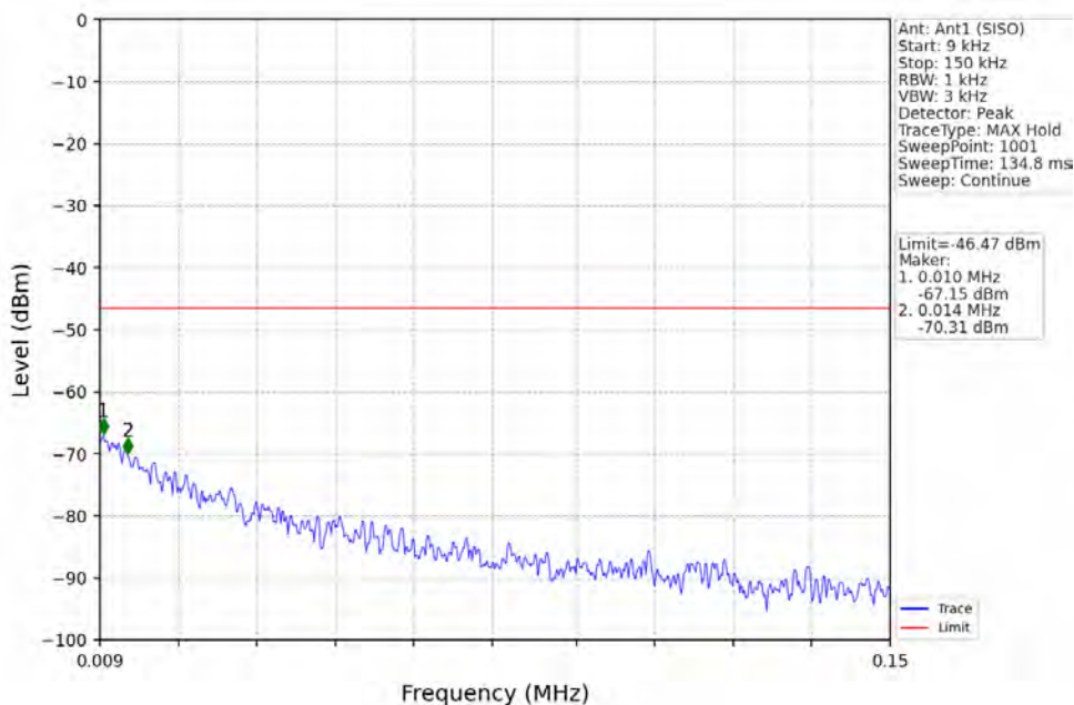
802.11ax(HEW20)_MCH_2437MHz_SU_Ant1 (SISO)_NTNV
