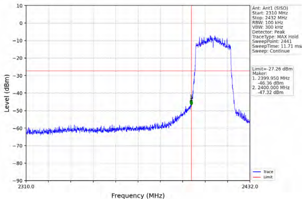
802.11ax(HEW20)_LCH_2412MHz_SU_Ant1 (SISO)_NTNV
