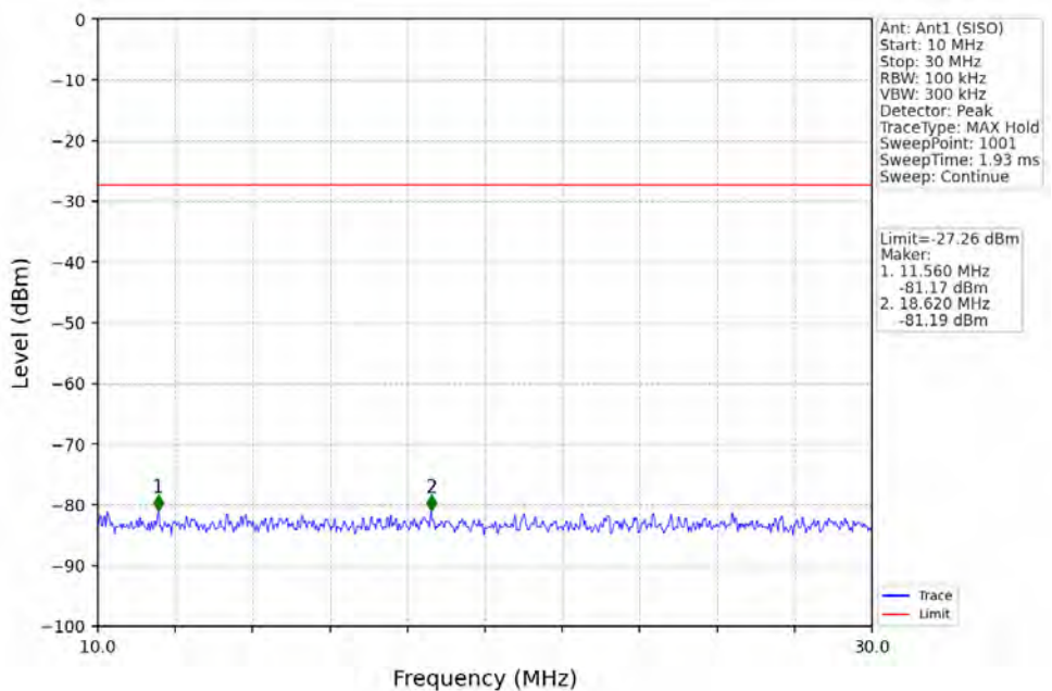
802.11ax(HEW20)_LCH_2412MHz_SU_Ant1 (SISO)_NTNV
