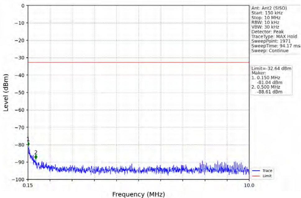
802.11ax(HEW20)_MCH_2437MHz_SU_Ant2 (SISO)_NTNV
