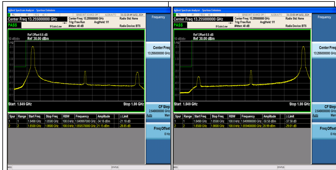
Band2_10MHz_QPSK_18650_1RB#0
