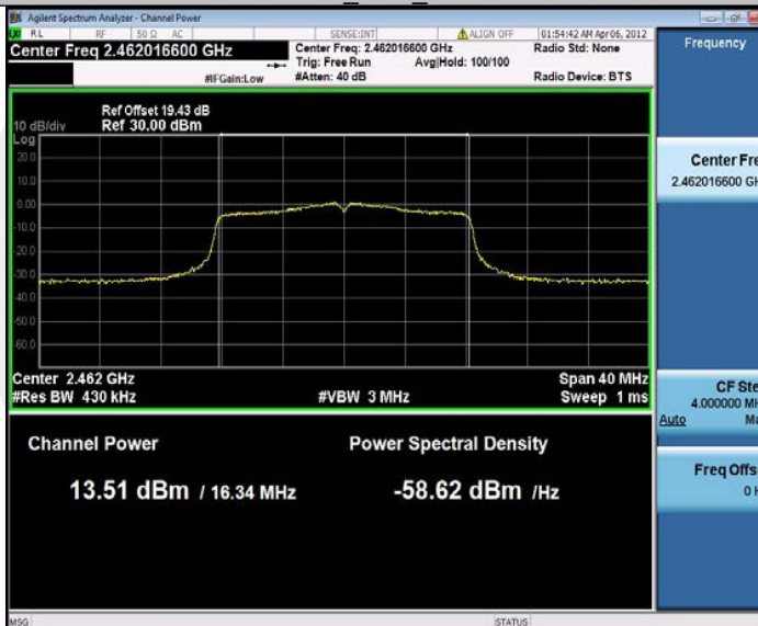
11G Ant2_2462
