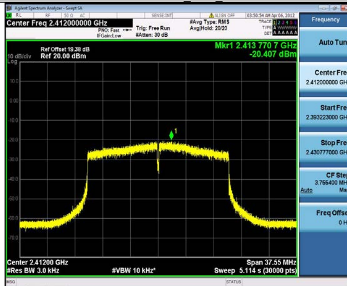
11AX20MIMO_Ant2_2412
