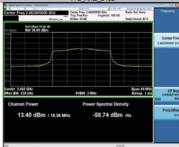
11G Ant2_2462
