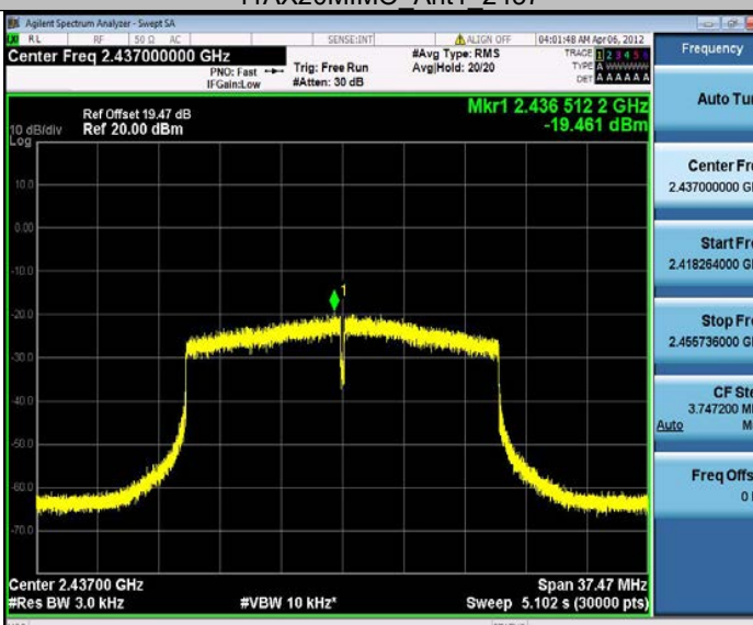
11AX20MIMO_Ant1_2437
