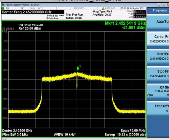
11AX40MIMO_Ant2_2452
