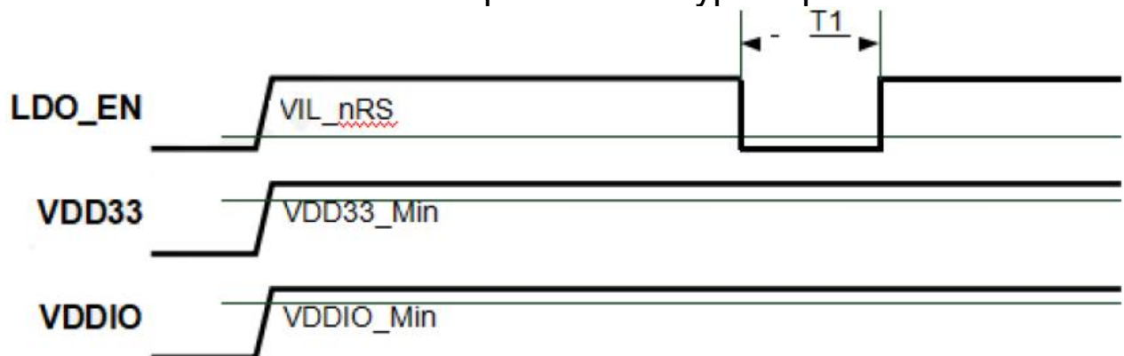
Reset Timing Parameters
