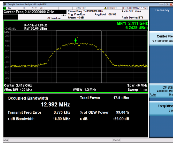
11B_Ant1_2412
