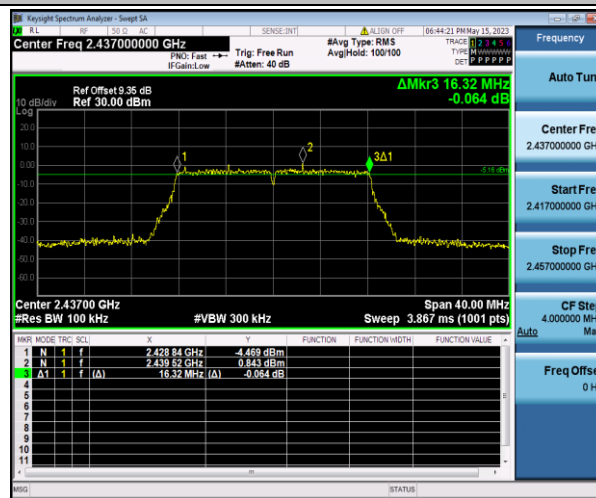
11G_Ant1_2437
