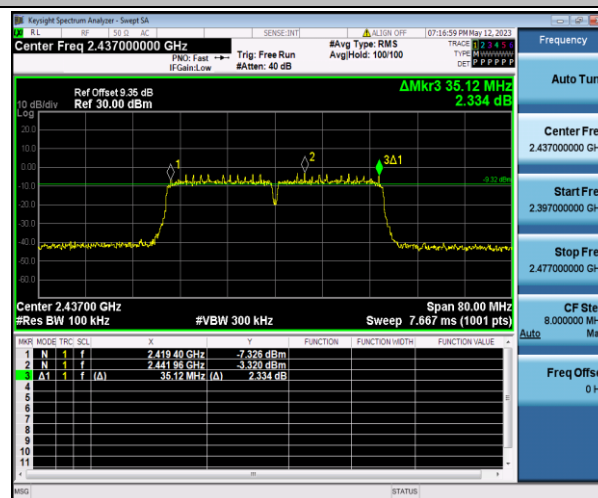
11N40SISO_Ant1_2437
