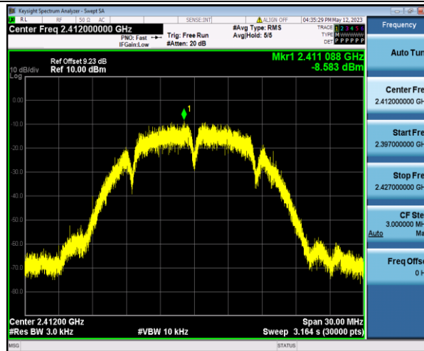
11B_Ant1_2412
