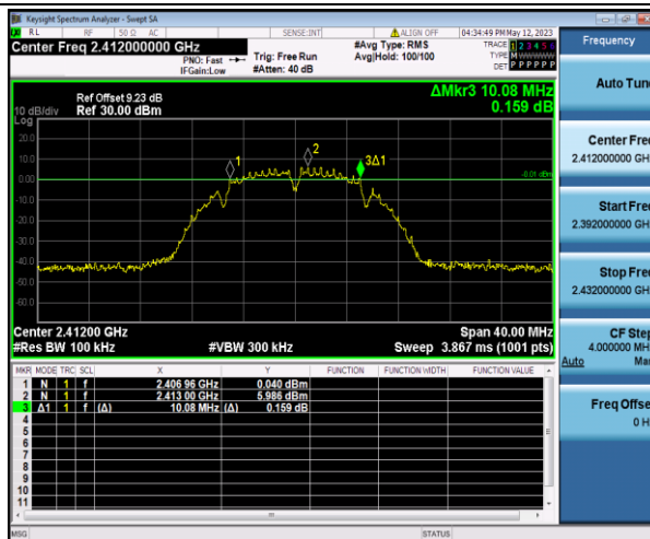
11B_Ant1_2412
