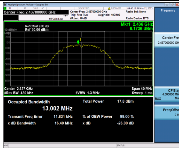
11B_Ant1_2437
