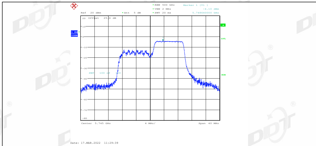
11AX20MIMO_Ant2_5745_26Tone_RU0
