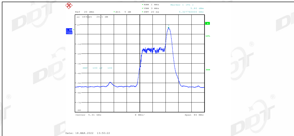
11AX40MIMO Ant1 5310 52Tone RU37
