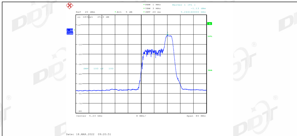
11AX40MIMO Ant1 5230 106Tone RU53
