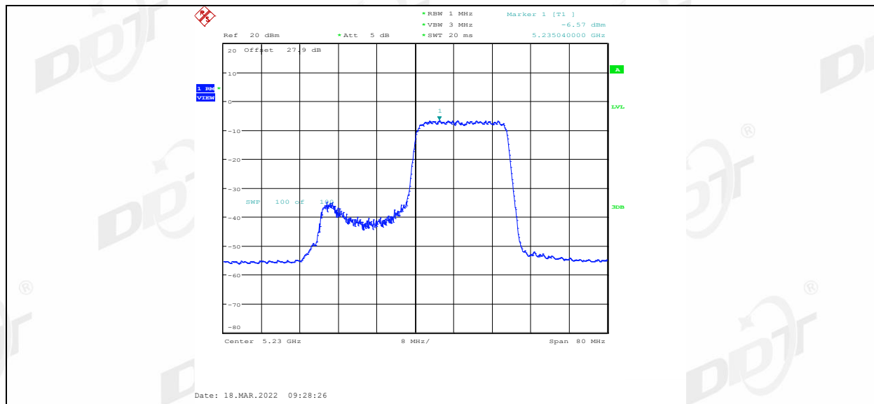
11AX40MIMO_Ant2_5230_26Tone_RU0
