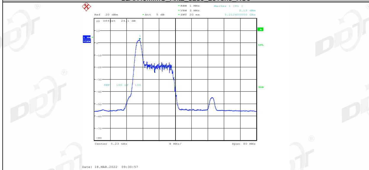
11AX40MIMO_Ant2_5230_26Tone_RU8
