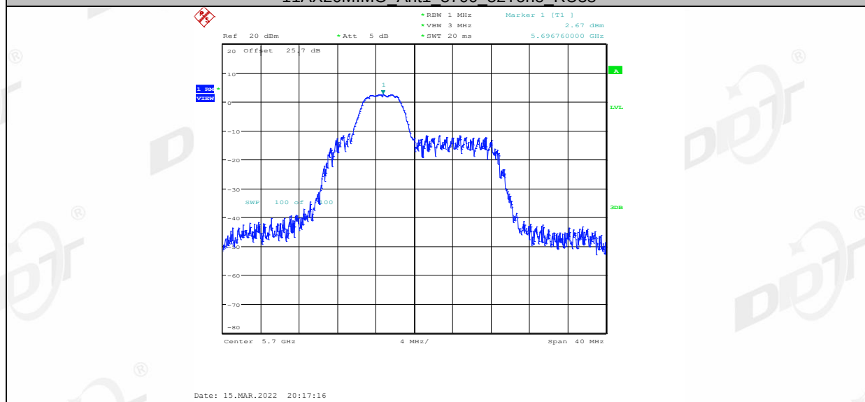
11AX20MIMO Ant1 5700 52Tone RU39
