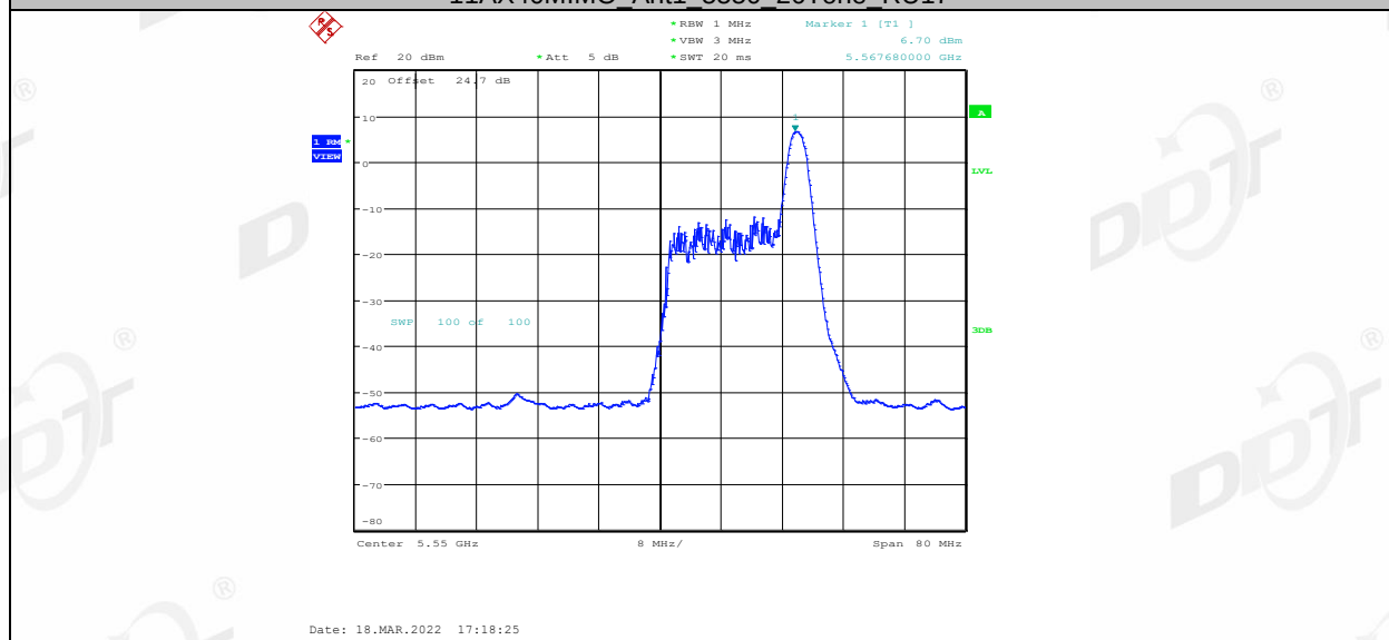
11AX40MIMO Ant1 5550 52Tone RU37
