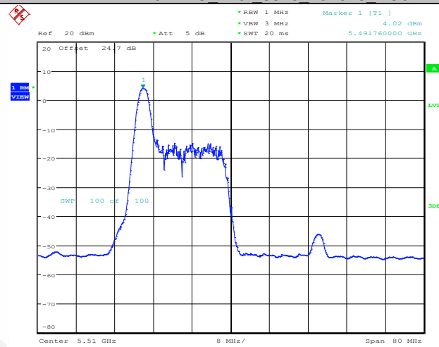
11AX40MIMO_Ant2_5510_26Tone_RU0
