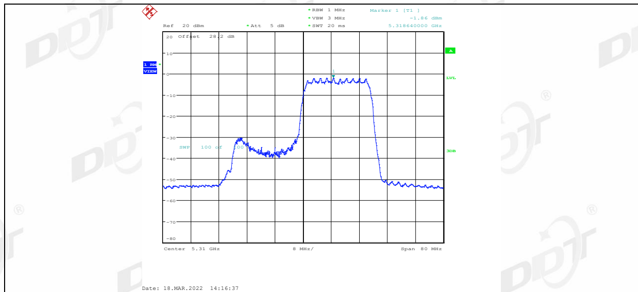
11AX40MIMO_Ant2_5310_26Tone_RU0
