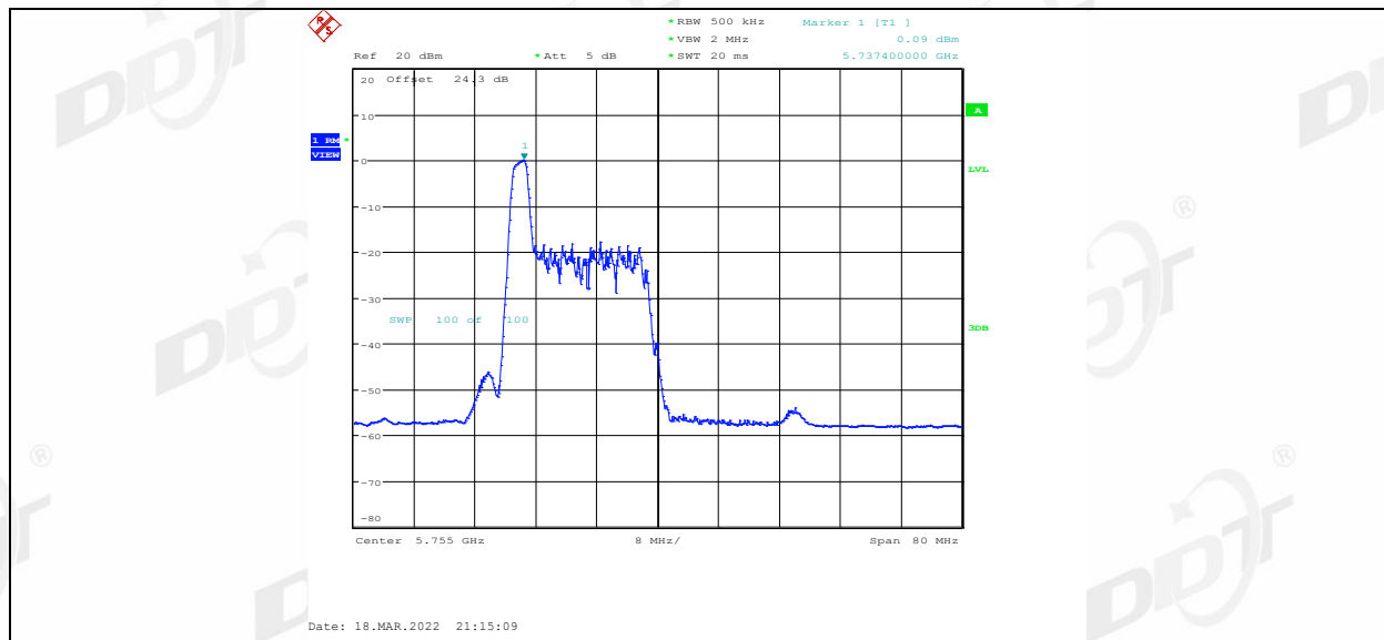
11AX40MIMO Ant1 5755 26Tone RU8
