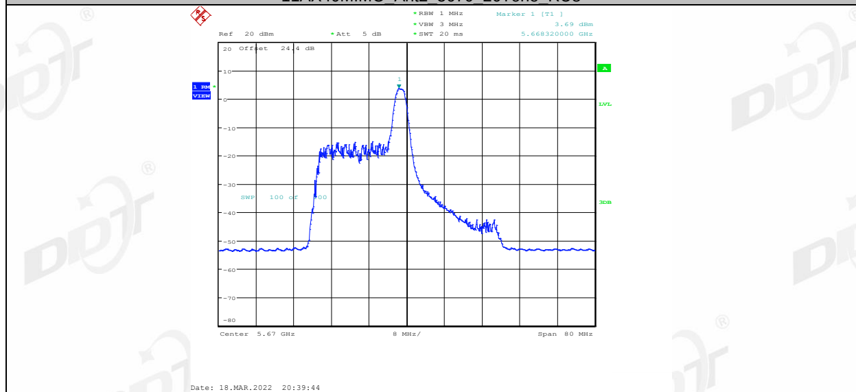
11AX40MIMO_Ant2_5670_26Tone_RU17
