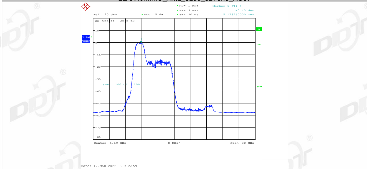
11AX40MIMO Ant1 5190 52Tone RU40
