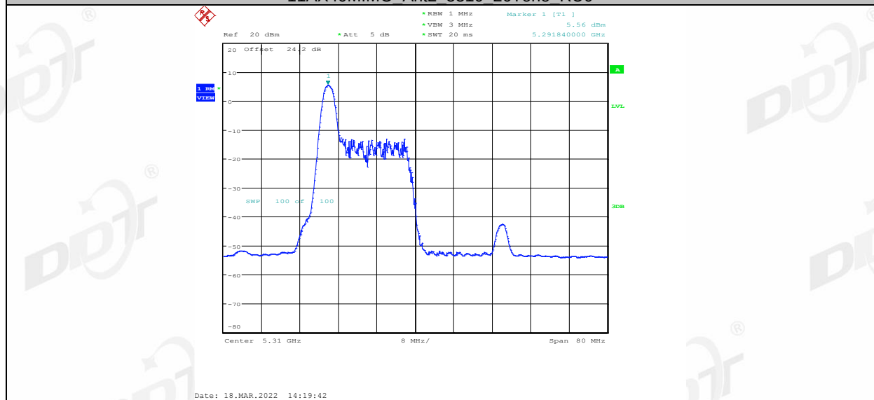
11AX40MIMO_Ant2_5310_26Tone_RU8
