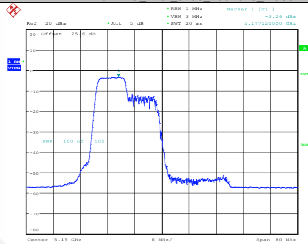
11AX40MIMO Ant1 5190 106Tone RU53
