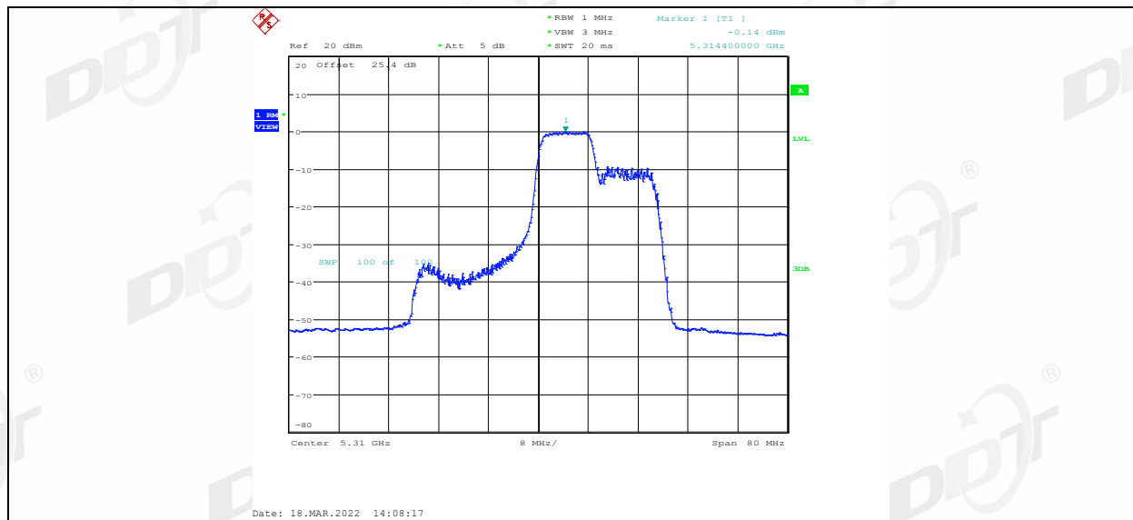
11AX40MIMO Ant1 5310 106Tone RU56
