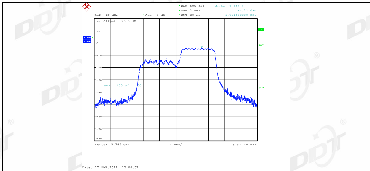
11AX20MIMO_Ant2_5785_26Tone_RU0
