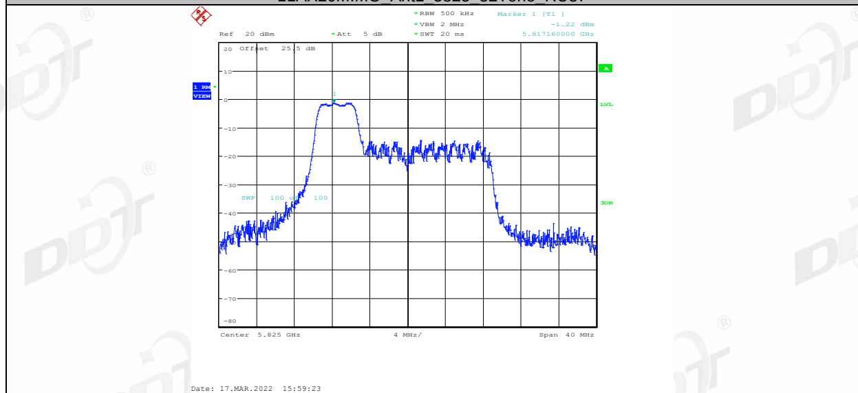
11AX20MIMO Ant1 5825 52Tone RU38
