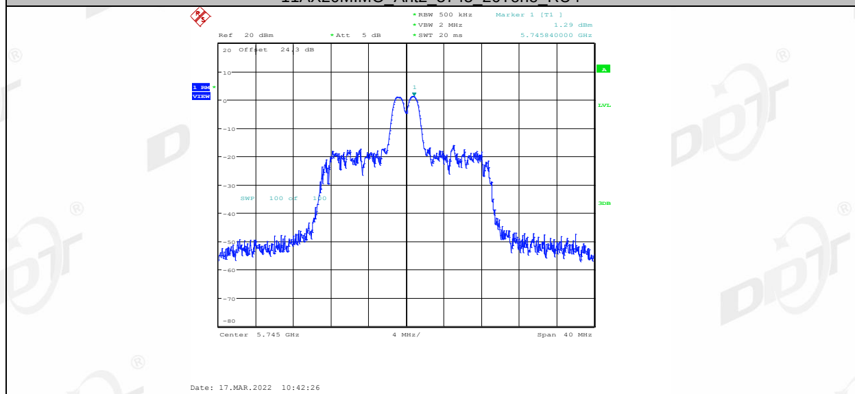
11AX20MIMO_Ant2_5745_26Tone_RU8
