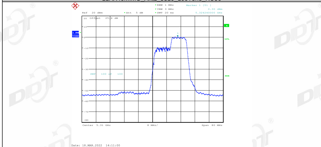
11AX40MIMO Ant1 5310 242Tone RU61
