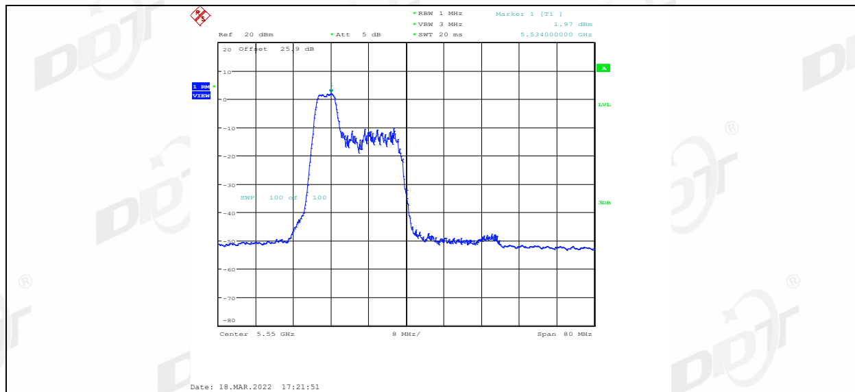
11AX40MIMO Ant1 5550 52Tone RU40
