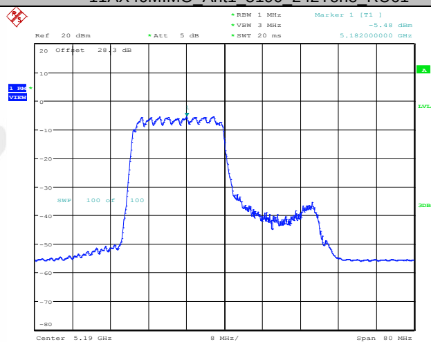
11AX40MIMO Ant1 5190 242Tone RU61
