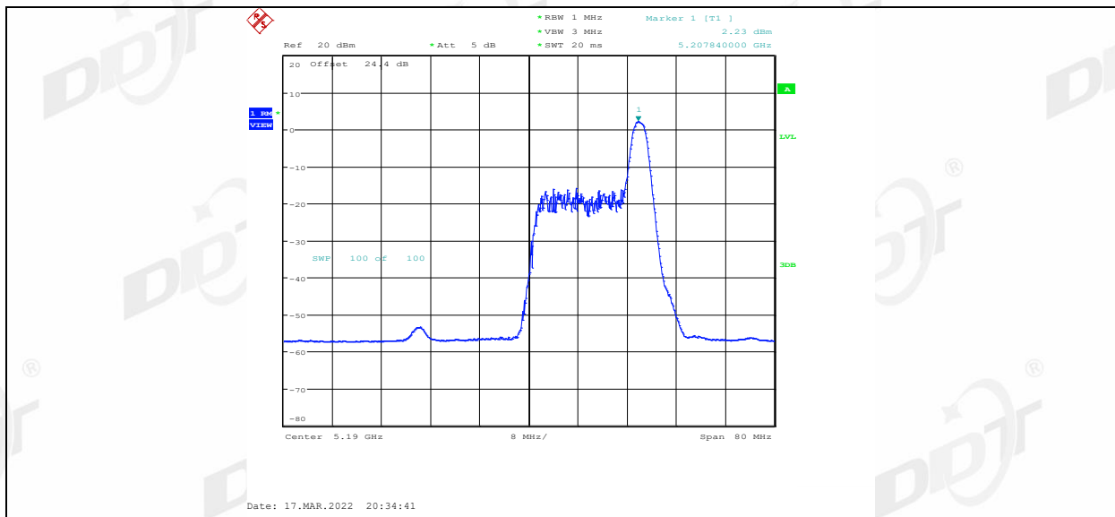
11AX40MIMO Ant1 5190 52Tone RU37
