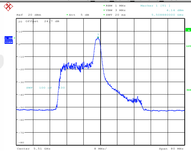
11AX40MIMO_Ant2_5510_26Tone_RU8
