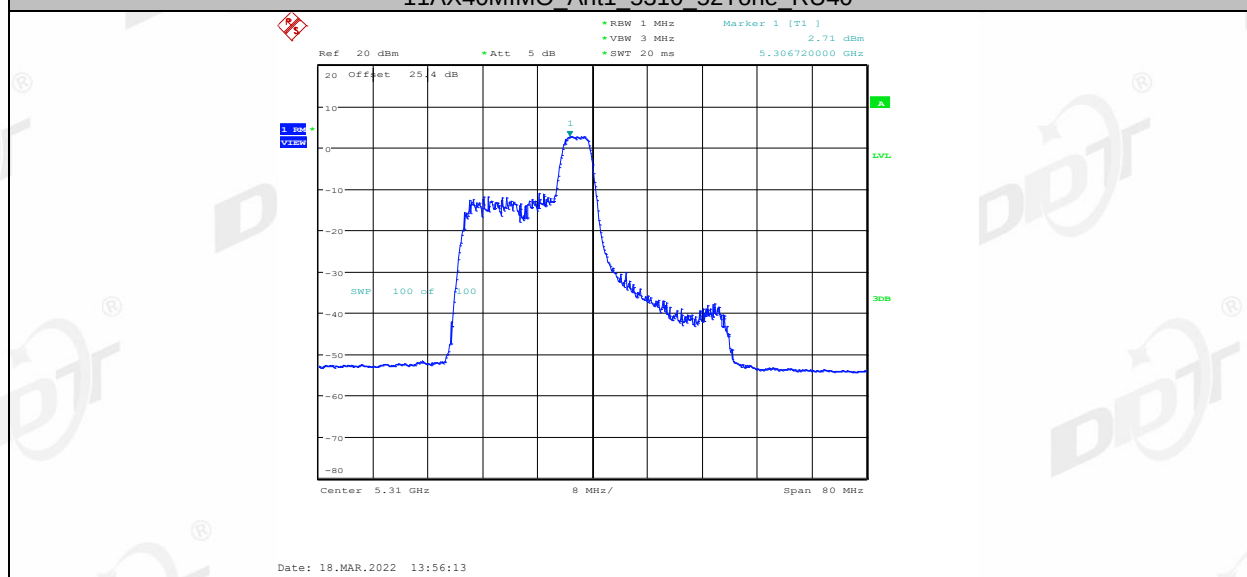
11AX40MIMO Ant1 5310 52Tone RU44
