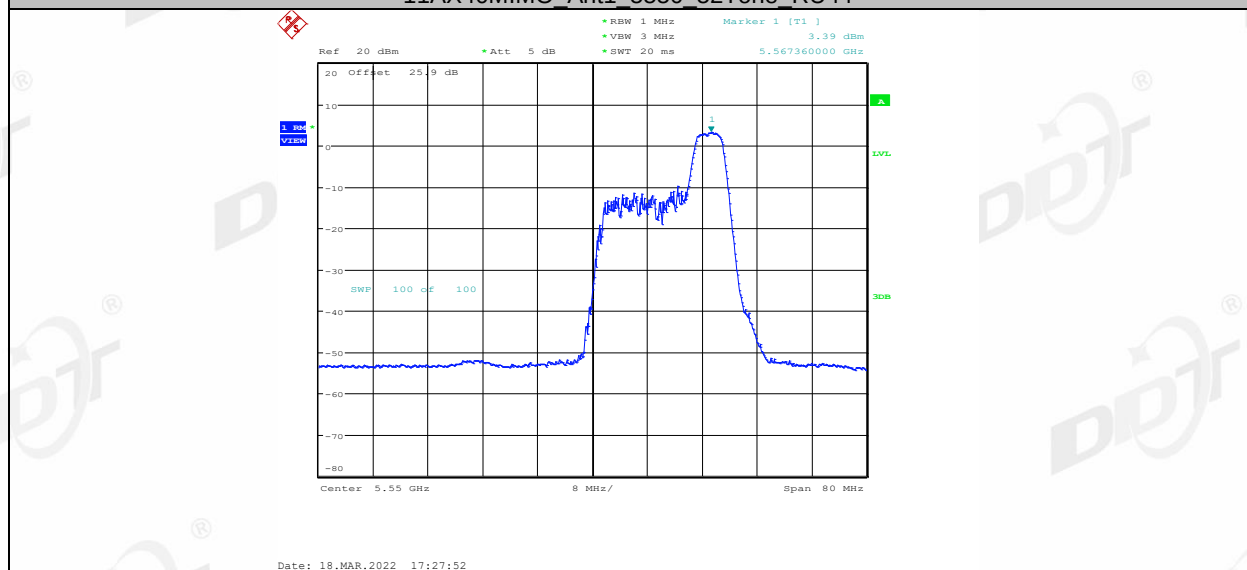
11AX40MIMO Ant1 5550 106Tone RU53
