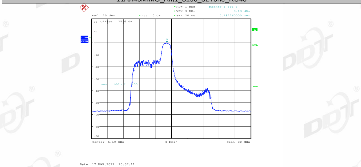
11AX40MIMO Ant1 5190 52Tone RU44
