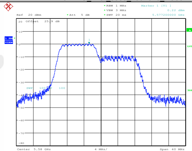
11AX20MIMO Ant1 5580 106Tone RU53
