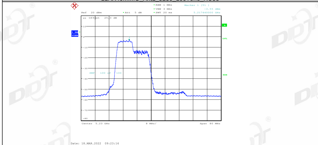
11AX40MIMO Ant1 5230 106Tone RU54
