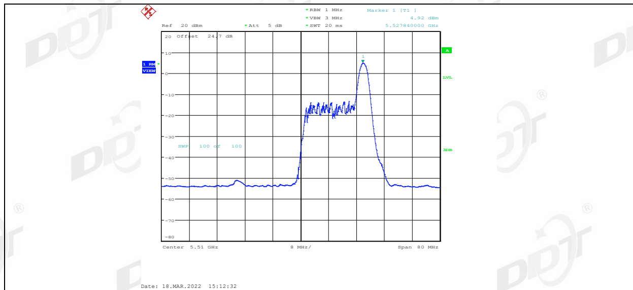
11AX40MIMO Ant1 5510 52Tone RU37
