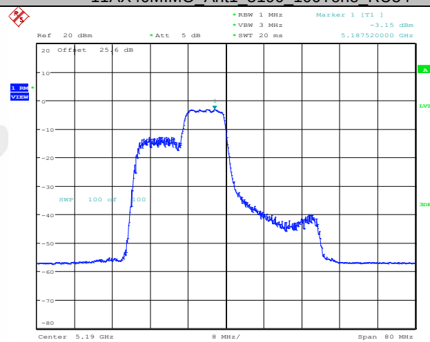
11AX40MIMO Ant1 5190 106Tone RU54
