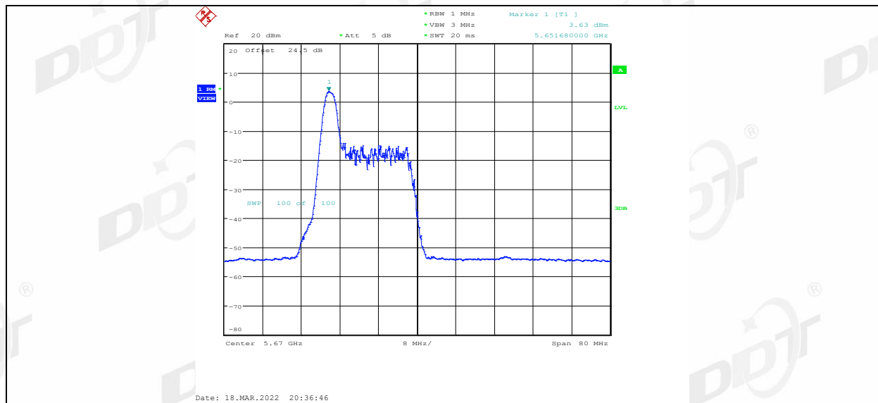
11AX40MIMO_Ant2_5670_26Tone_RU8
