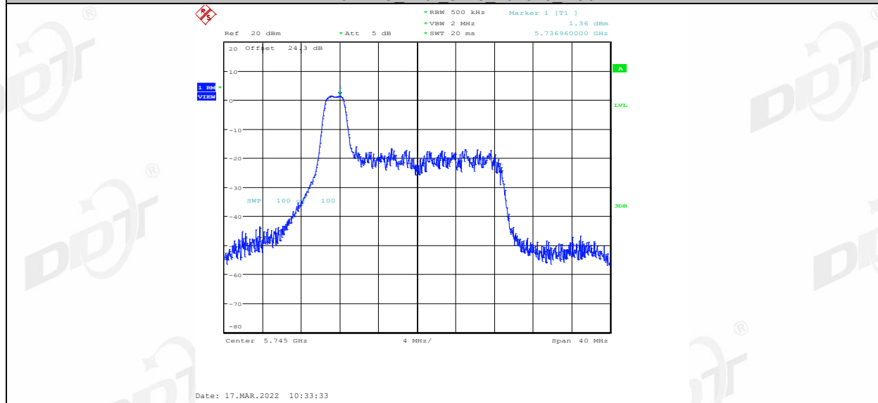
11AX20MIMO_Ant2_5745_26Tone_RU4
