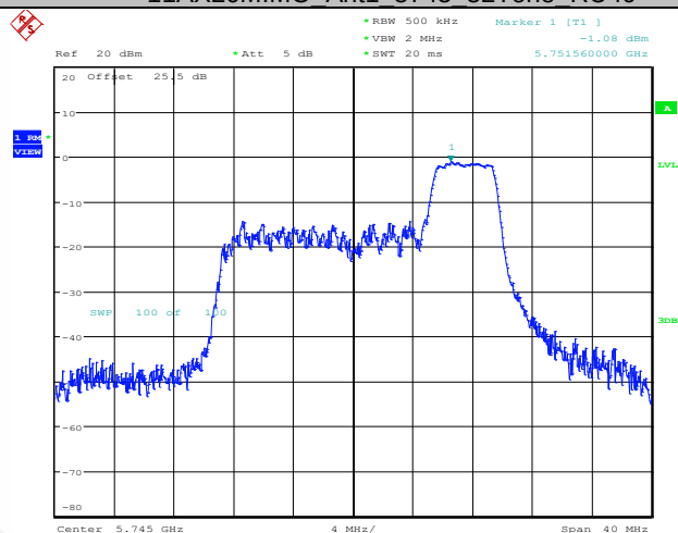
11AX20MIMO Ant1 5745 52Tone RU40
