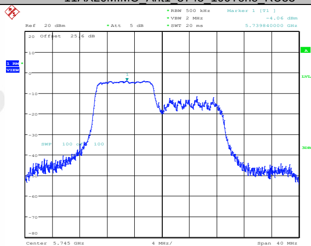
11AX20MIMO Ant1 5745 106Tone RU53
