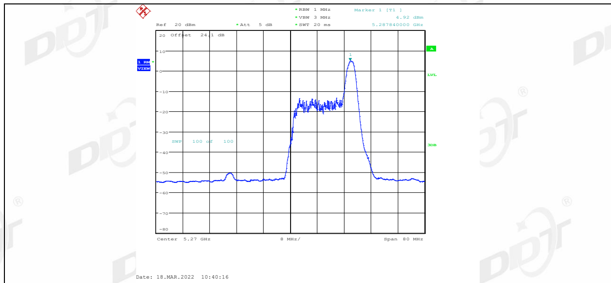
11AX40MIMO Ant1 5270 52Tone RU37
