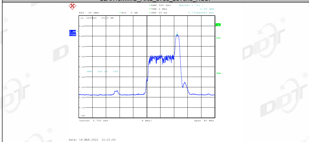
11AX40MIMO Ant1 5755 52Tone RU37
