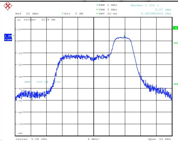
11AX20MIMO_Ant1_5580_52Tone_RU40
