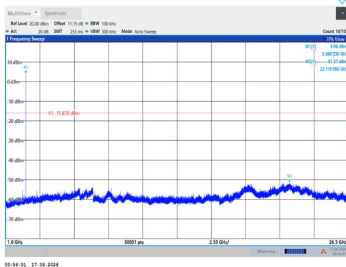
BLE_1M_Ant1_2480_1000~26500
