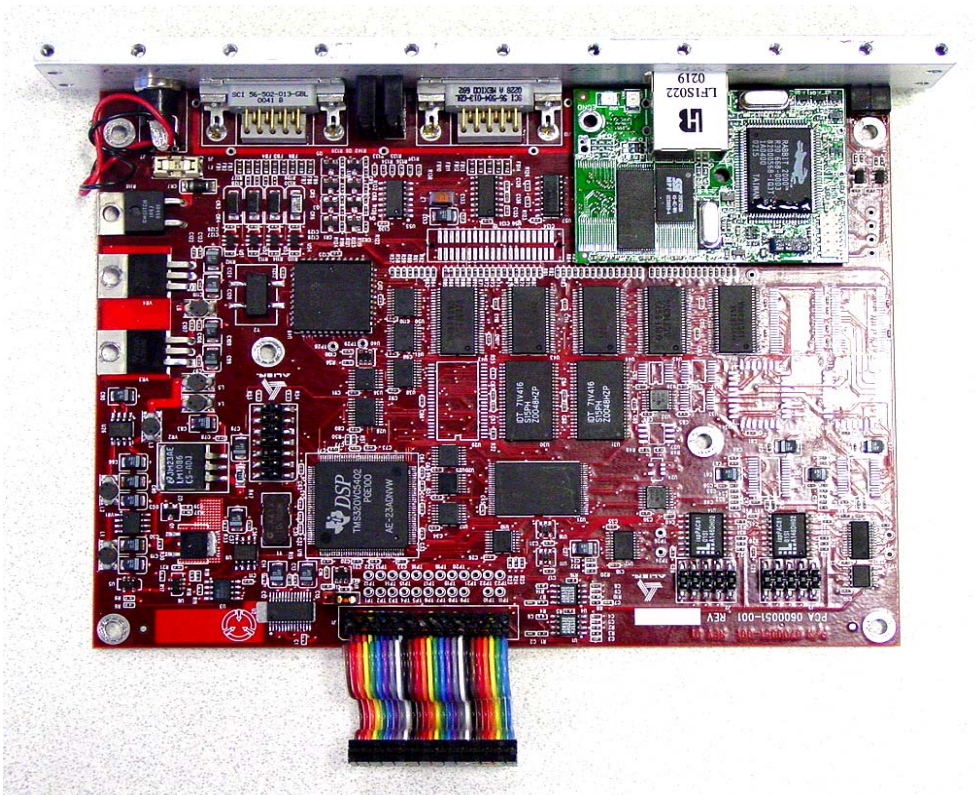
Microprocessor PCA Top
