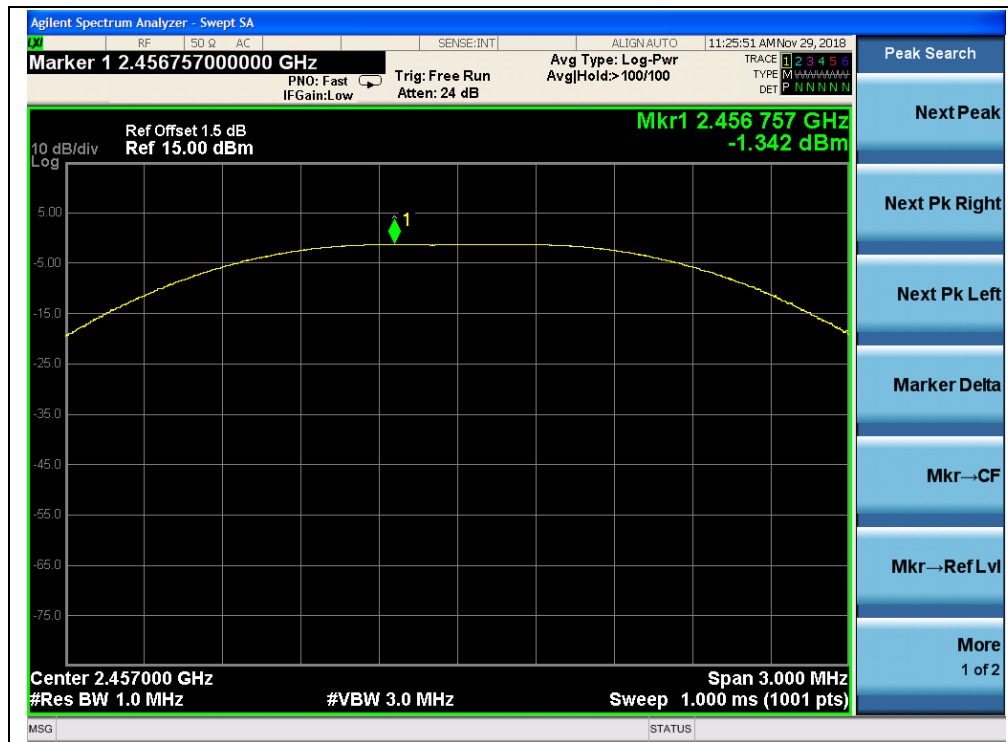
(Power_2457MHz)
