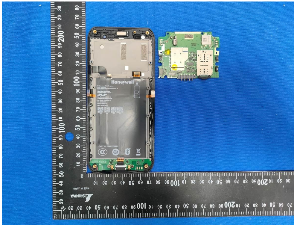
(9) EUT Photo
