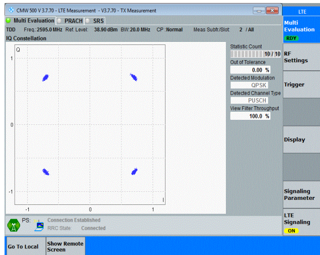
Band41-20MHz-QPSK-40640-100RB#0
