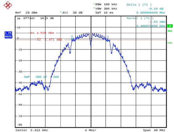
b_2412MHz_Chain 1 9.600MHz
