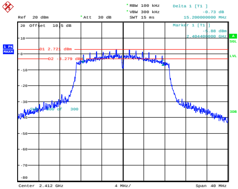
n20_2412MHz_Chain 0 15.200MHz
