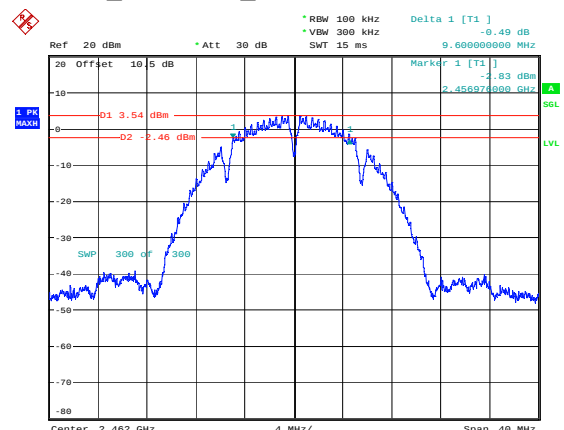
b_2462MHz_Chain 1 9.600MHz
