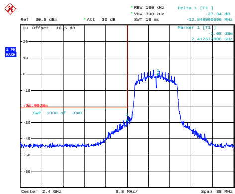
n20_2412MHz_Chain 0 27.34dB
