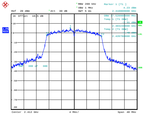
n20_2412MHz_Chain 0 17.520MHz
