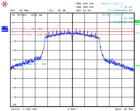
n20_2462MHz_Chain 0 15.200MHz
