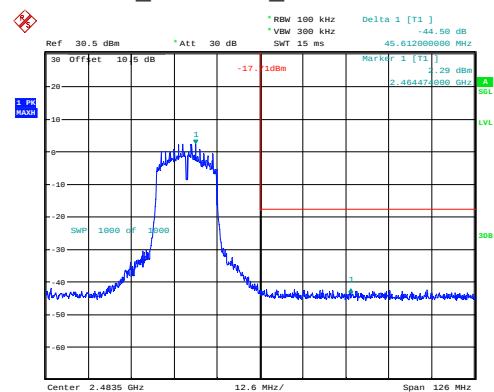
n20_2462MHz_Chain 1 44.50dB
