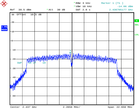
g_2437MHz_Chain 1 -14.06dBm/3kHz
