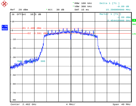
n20_2462MHz_Chain 1 15.200MHz
