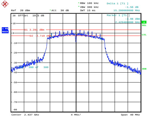
n20_2437MHz_Chain 0 15.200MHz
