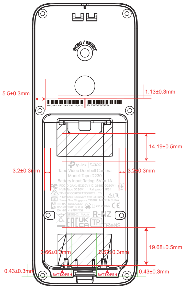
尺寸图
