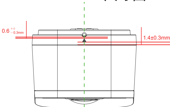
尺寸图
