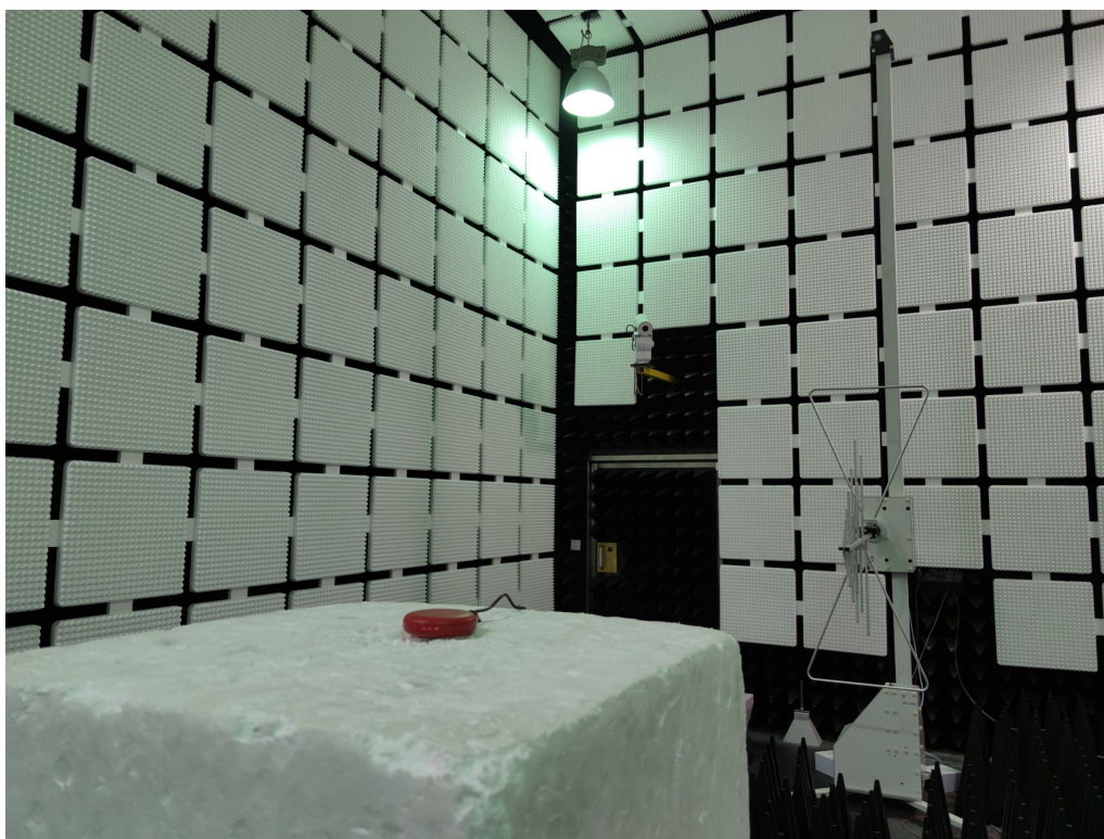
Fig. 2 (Above 1GHz)
