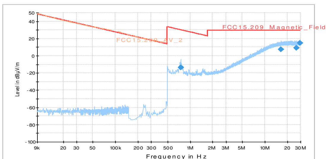
FCC15.209_magn hor+vert
