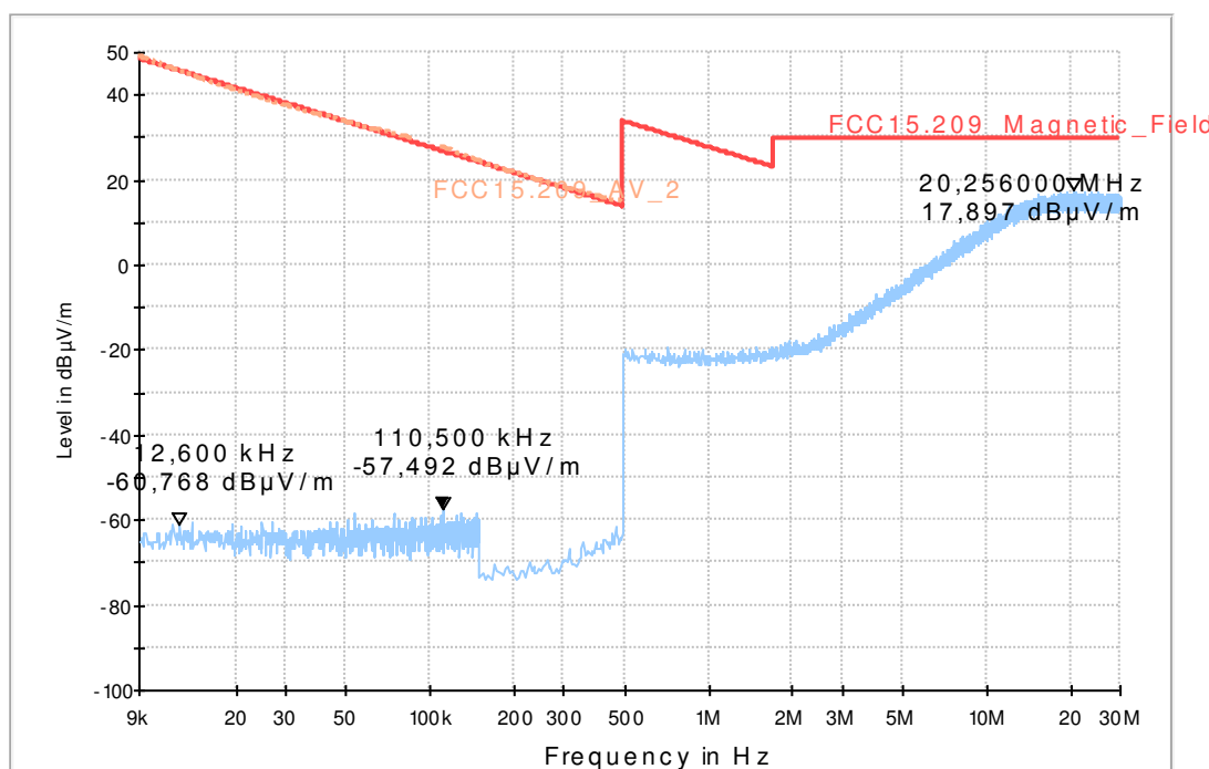
FCC15.209_magn hor+vert
