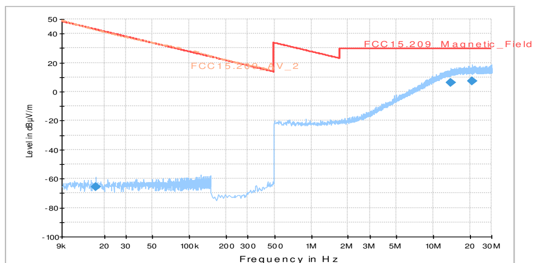
FCC15.209_magn hor+vert
