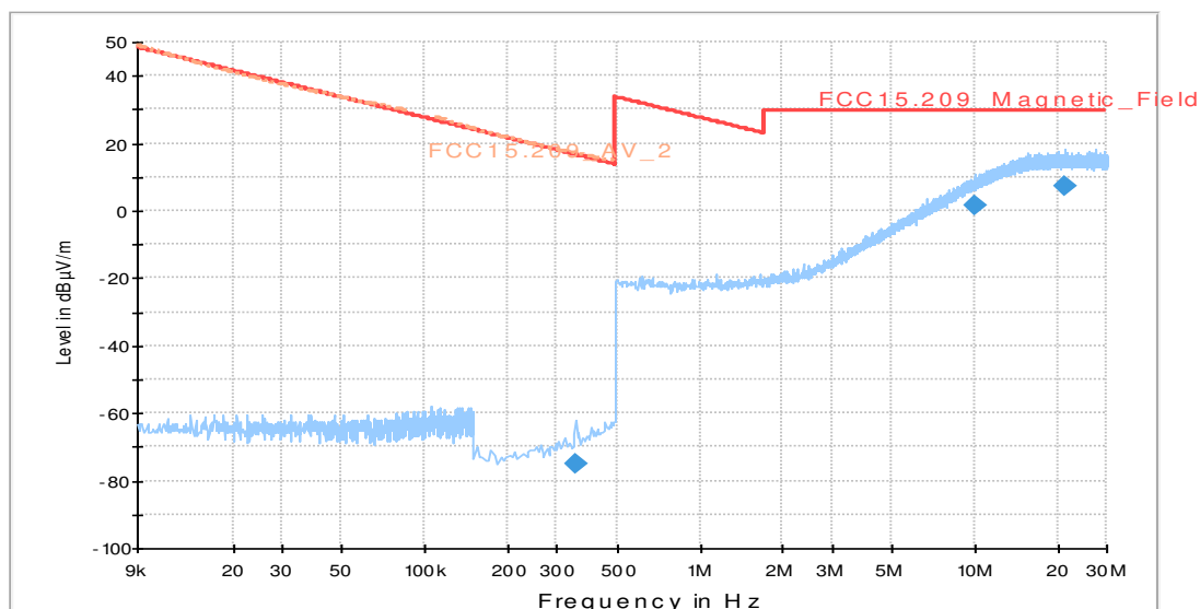
FCC15.209_magn hor+vert
