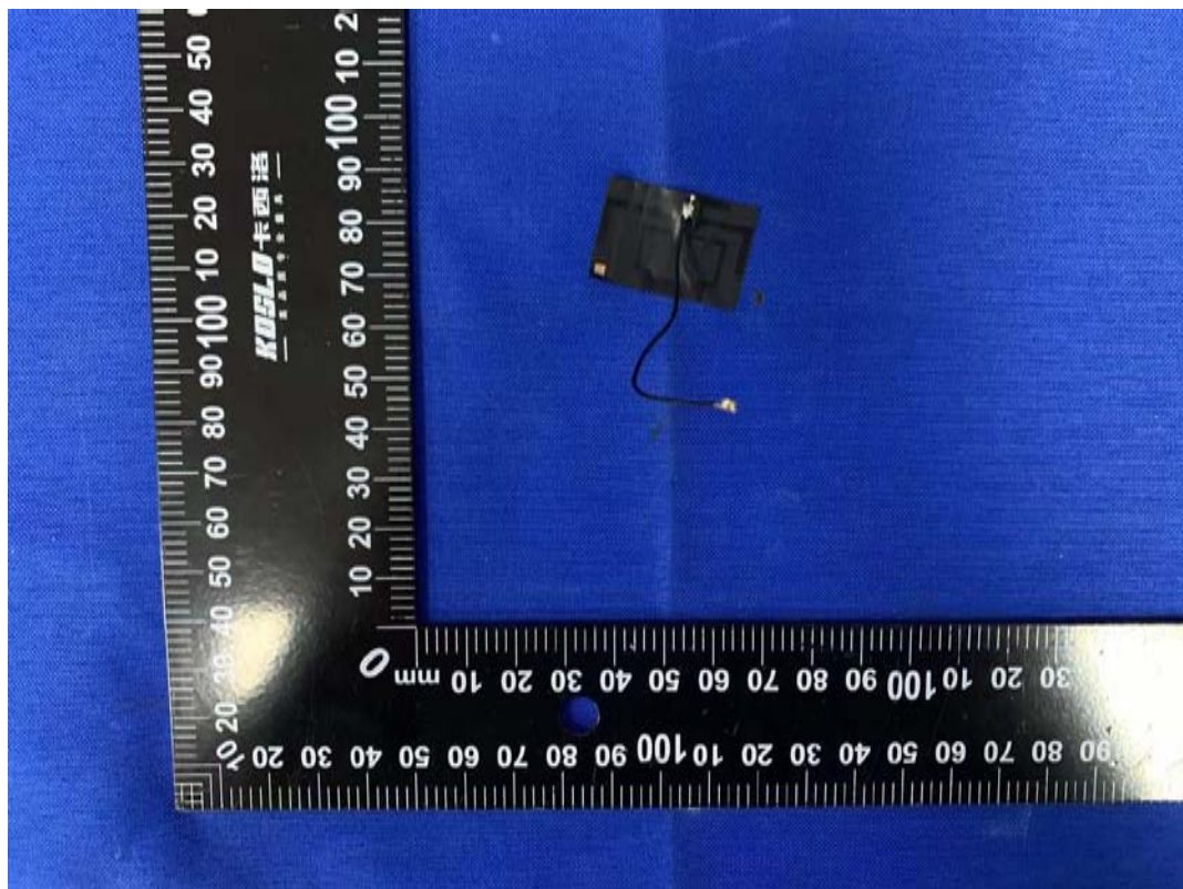
5.8G Antenna
