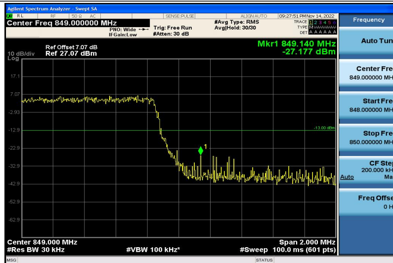
Band5-3MHz-QPSK-20635-15RB#0
