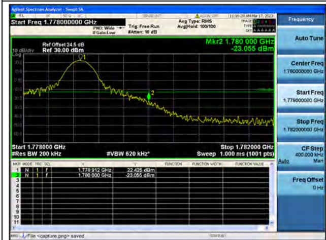
Band66 / 20MHz / High CH / QPSK / 1 RB
