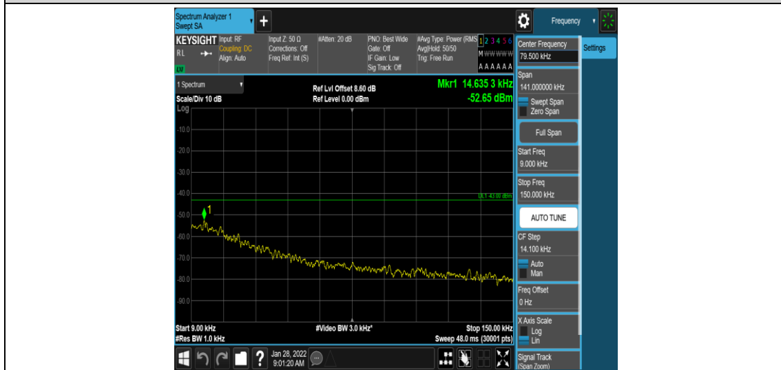
Band4-20MHz-QPSK-20050-1-0-Low-0.009-0.15--52.65-PASS
