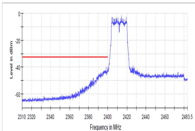
Band Edge
