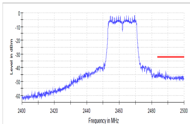
Band Edge
