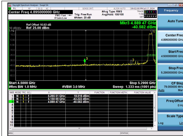
11AC20MIMO-Ant0-5320-PASS
