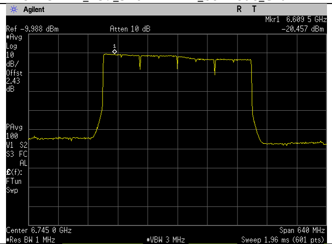
6745MHz_159_320MHz BW_be-mode_Chain 3
