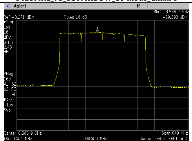
6585MHz_127_320MHz BW_be-mode_Chain 1
