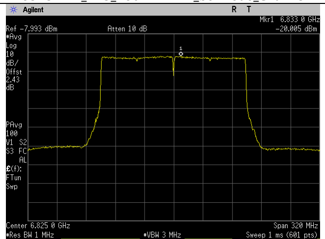
6825MHz_175_160MHz BW_be-mode_Chain 1
