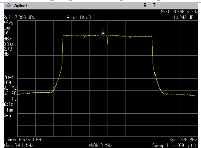
6575MHz_143_160MHz BW_be-mode_Chain 1
