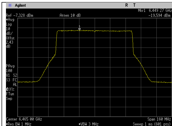
6465MHz_103_80MHz BW_be-mode_Chain 0
