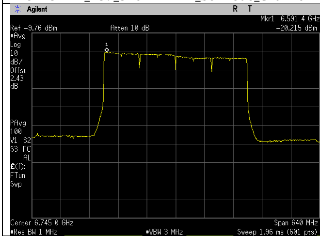
6745MHz_159_320MHz BW_be-mode_Chain 2
