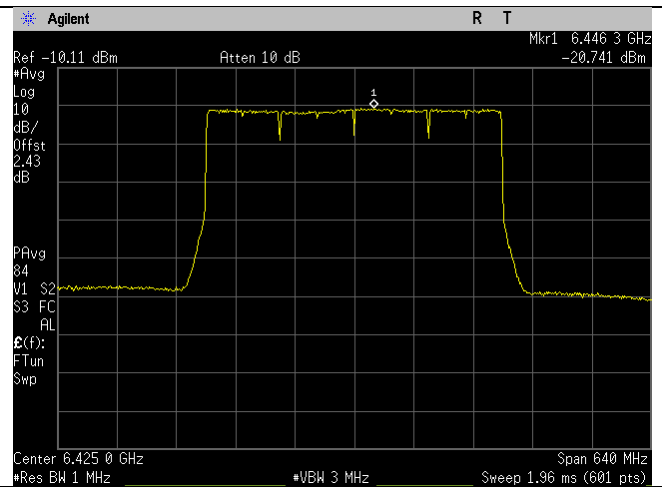
6425MHz_95_320MHz BW_be-mode_Chain 1
