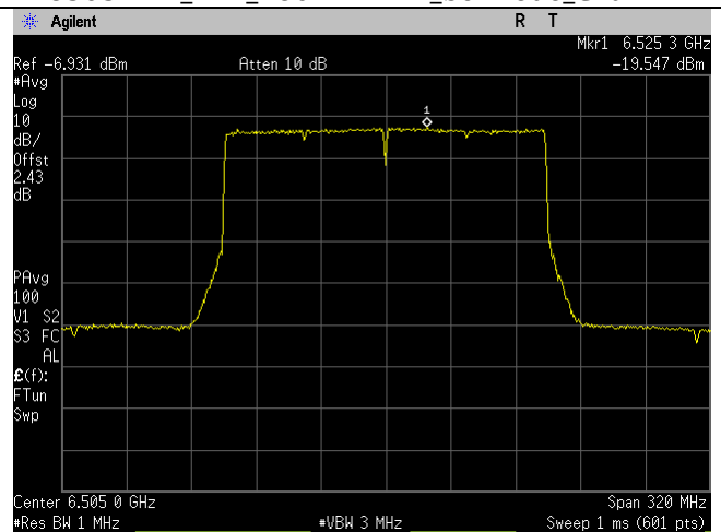
6505MHz_111_160MHz BW_be-mode_Chain 3
