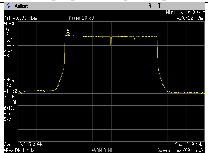
6825MHz_175_160MHz BW_be-mode_Chain 3
