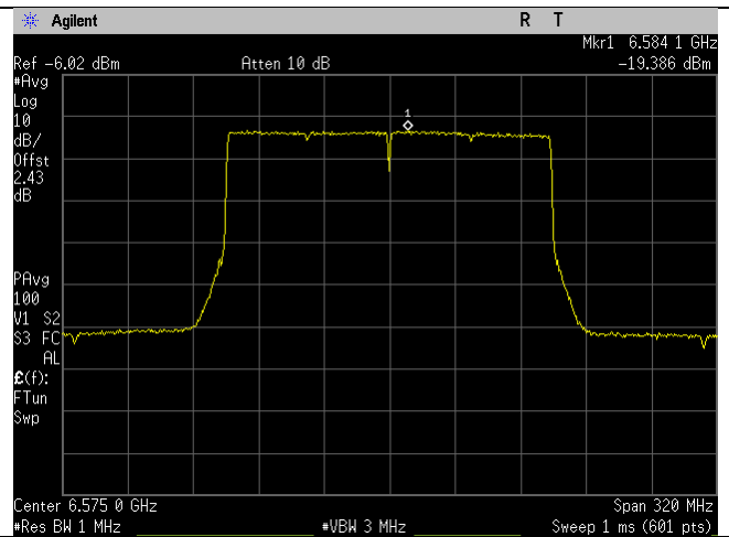
6575MHz_143_160MHz BW_be-mode_Chain 3
