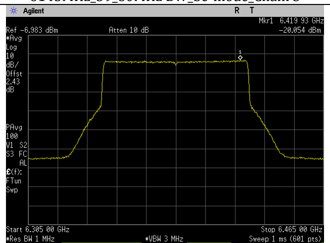
6385MHz_87_80MHz BW_be-mode_Chain 1
