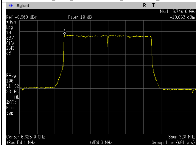
6825MHz_175_160MHz BW_be-mode_Chain 2
