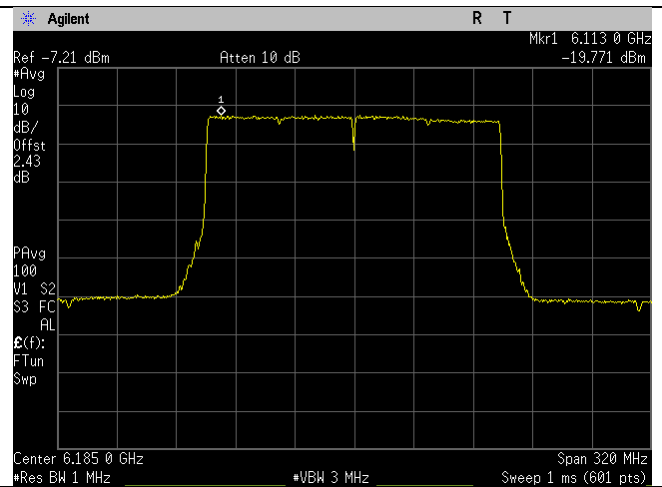
6185MHz_47_160MHz BW_be-mode_Chain 3
