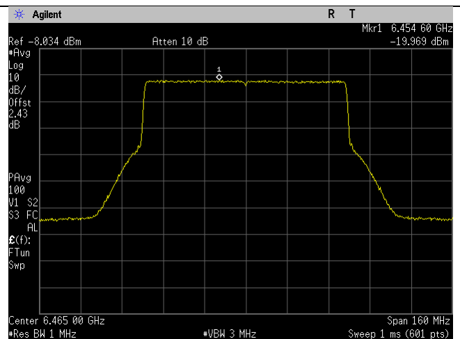
6465MHz_103_80MHz BW_be-mode_Chain 1
