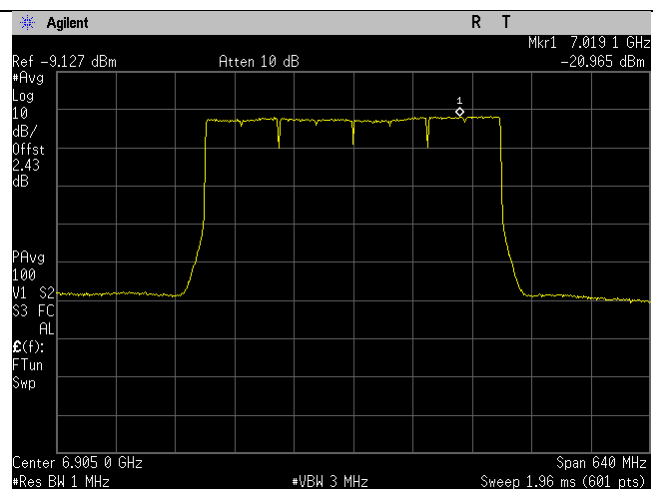
6905MHz_191_320MHz BW_be-mode_Chain 1
