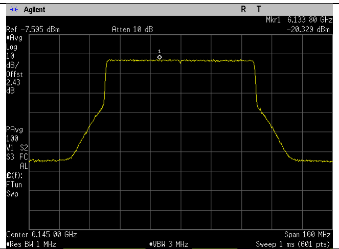
6145MHz_39_80MHz BW_be-mode_Chain 3
