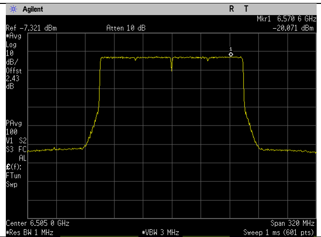
6505MHz_111_160MHz BW_be-mode_Chain 1
