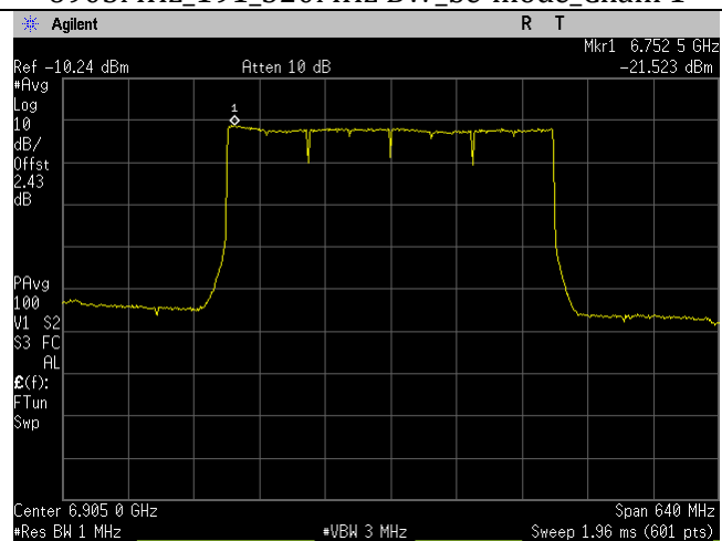
6905MHz_191_320MHz BW_be-mode_Chain 3
