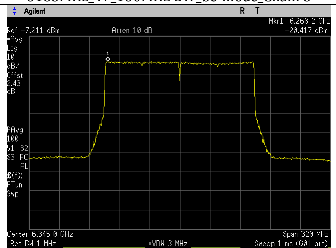
6345MHz_79_160MHz BW_be-mode_Chain 1
