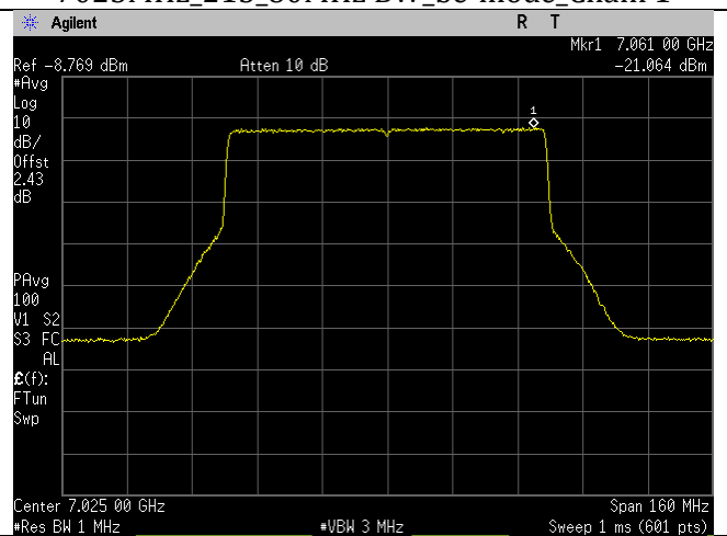
7025MHz_215_80MHz BW_be-mode_Chain 3
