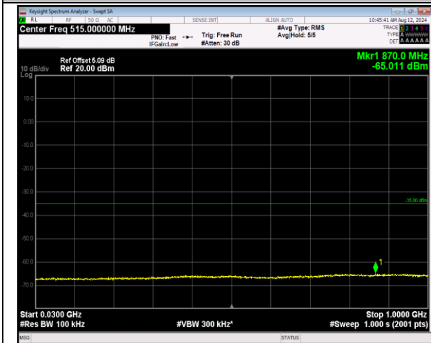
7-7-10MHz-20MHz-QPSK-QPSK-21006-21150-50RB#0-1 00RB#0-30~1000MHz-PASS
