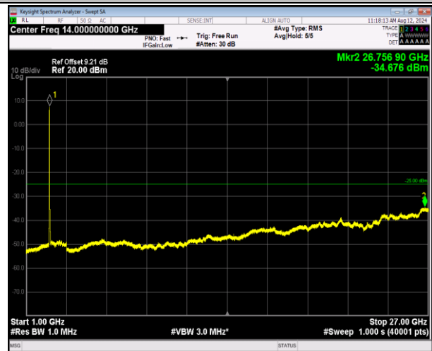
7-7-20MHz-10MHz-QPSK-QPSK-20850-20994-100RB#0-50RB#0-1000~27000MHz-PASS
