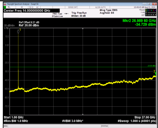
7-7-10MHz-20MHz-QPSK-QPSK-21206-21350-1RB#0-1RB #99-1000~27000MHz-PASS
