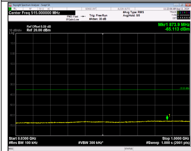
7-7-20MHz-10MHz-QPSK-QPSK-21051-21195-100RB#0- 50RB#0-30~1000MHz-PASS
