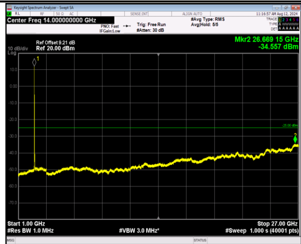
7-7-20MHz-10MHz-QPSK-QPSK-20850-20994-1RB#0-1RB #49-1000~27000MHz-PASS
