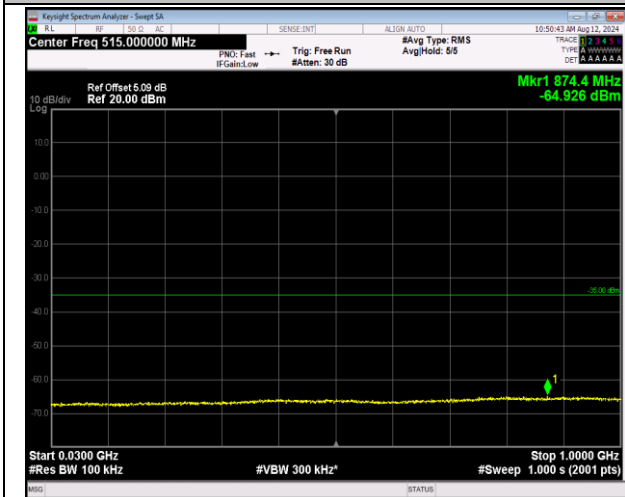
7-7-10MHz-20MHz-QPSK-QPSK-21206-21350-50RB#0-100RB#0-30~1000MHz-PASS
