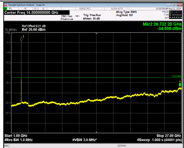
7-7-10MHz-20MHz-QPSK-QPSK-21206-21350-50RB#0-100RB#0-1000~27000MHz-PASS
