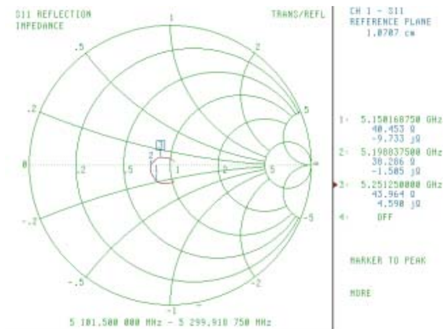
第一圖面：史密斯阻抗圖
