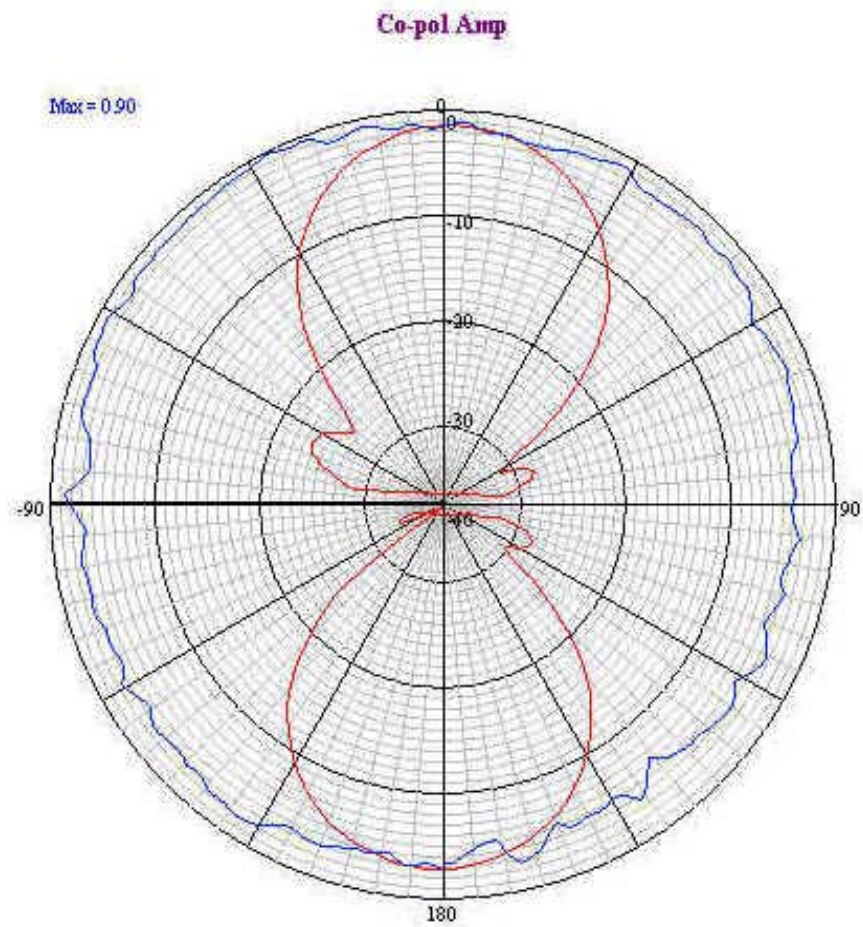
第三圖面：天線輻射場型
