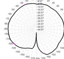
2500.0MHz Total(E2-YZ), Max=-6.70dB
