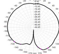
2490.0MHz Total(E2-YZ), Max=-6.45dB
