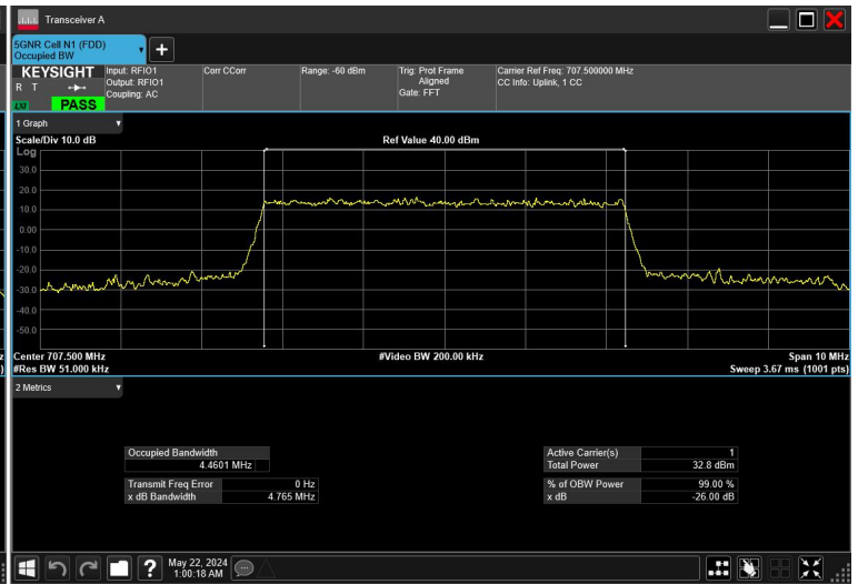
5MHz_15kHz_707.5MHz_DFT-s-OFDM QPSK_RB25@0
