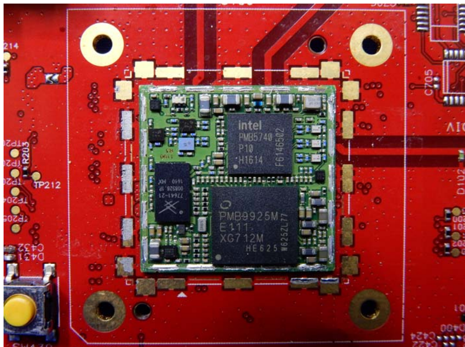
(4) EUT Photo
