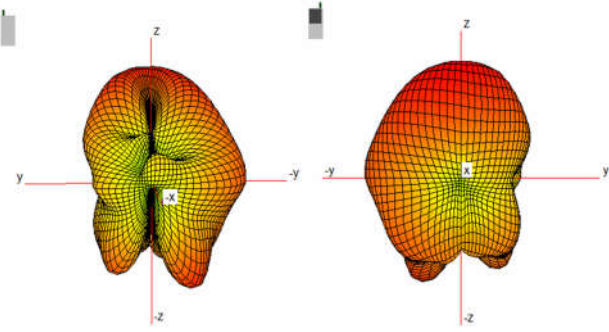
WIFI 6E (6100 MHz)
