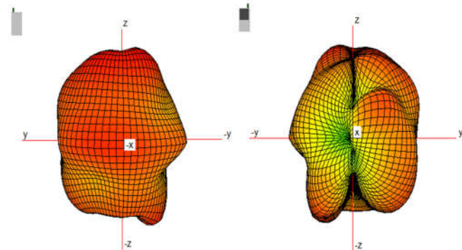
WIFI 6E (6100 MHz)
