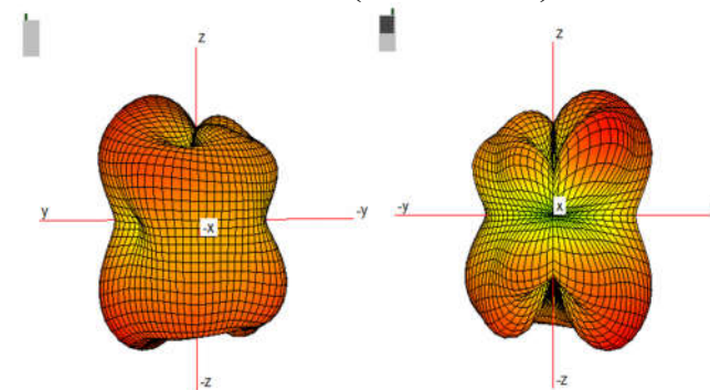
WIFI 6E (6700 MHz)
