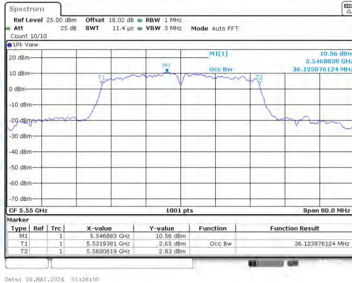
11N40MIMO_Ant2_5550
