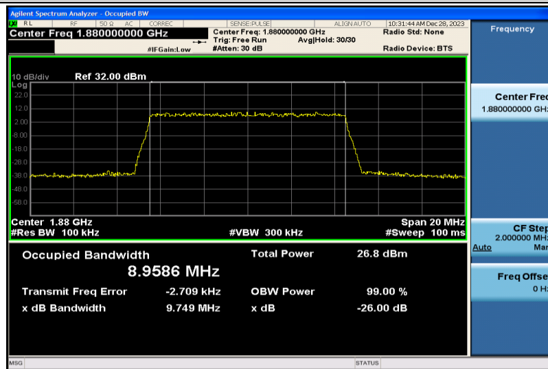
Band2-10MHz-QPSK-18900-50RB#0-8.9586
