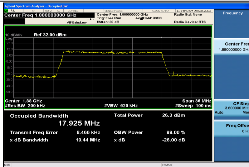
Band2-20MHz-QPSK-18900-100RB#0-17.925
