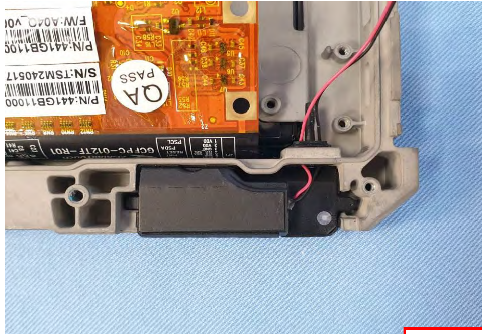
EUT Photo (66)
