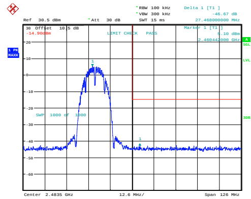
b_2462MHz_Chain 0 46.67dB
