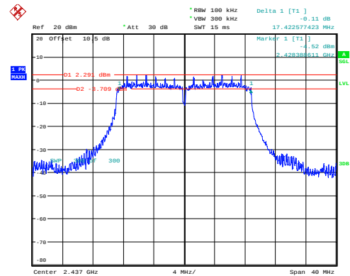
n20_2437MHz_Chain 0 17.423MHz
