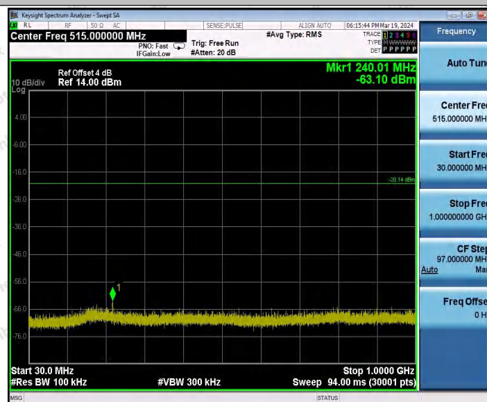
11AX40MIMO_Ant2_2422_30~1000
