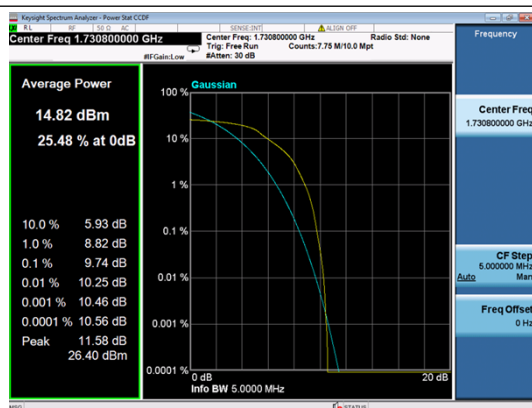
B4-5M-Mid CH-PAR-Q16
