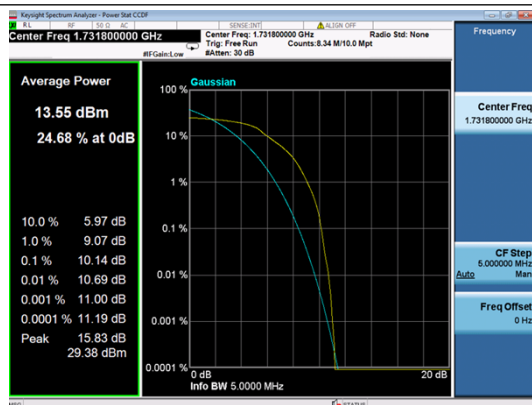
B4-5M-Mid CH-PAR-Q16
