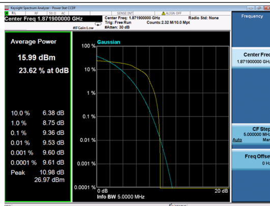
B2-20M-Mid CH-PAR-Q16
