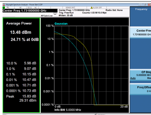
B4-5M-Mid CH-PAR-QPSK
