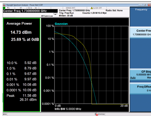
B4-5M-Mid CH-PAR-QPSK
