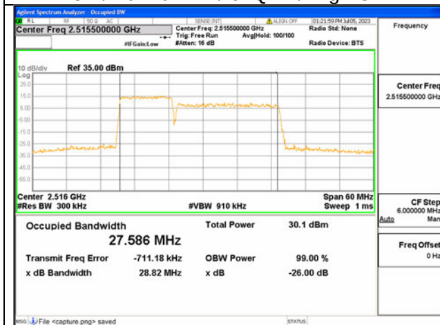
7C / 10+20MHz / QPSK/ Low CH
