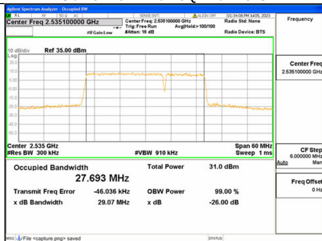
7C / 20+10MHz / QPSK/ Mid CH
