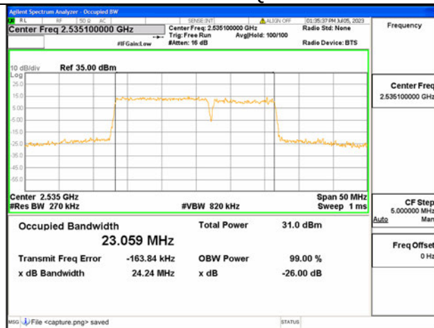
7C / 15+10MHz / 16QAM/ Mid CH
