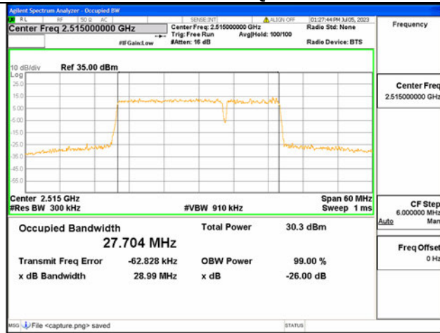
7C / 20+10MHz / 16QAM/ Low CH
