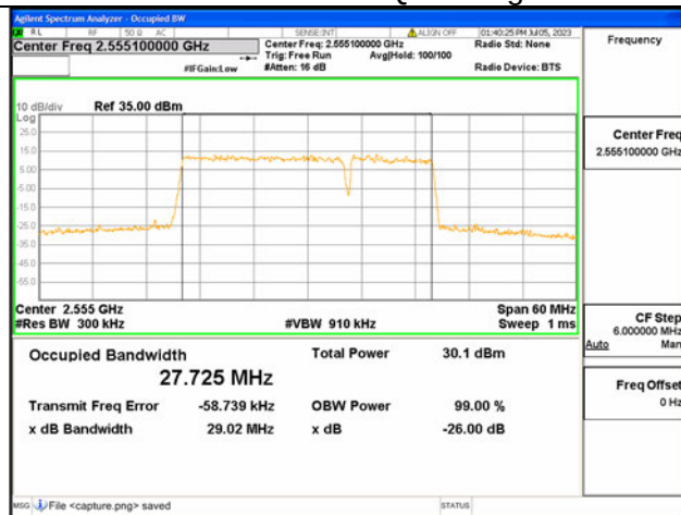
7C / 20+10MHz / 16QAM/ High CH
