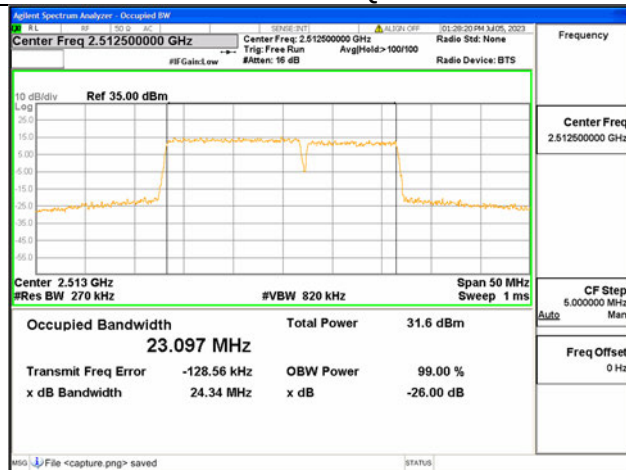
7C / 15+10MHz / QPSK/ Low CH
