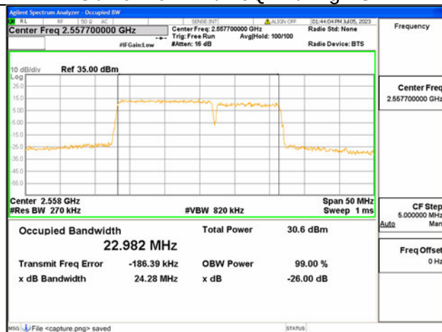
7C / 15+10MHz / QPSK/ High CH
