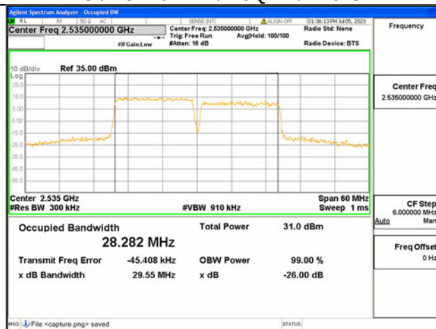
7C / 15+15MHz / QPSK/ Mid CH
