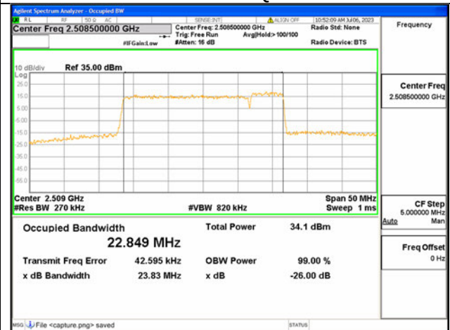
41C / 20+5MHz / QPSK/ Low CH
