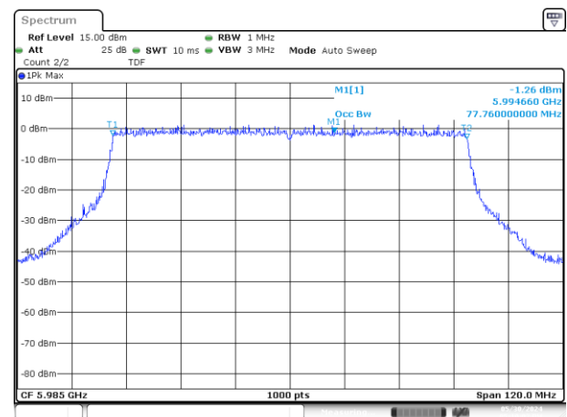
SISO-A 802.11ax/be80 ch7 99%
