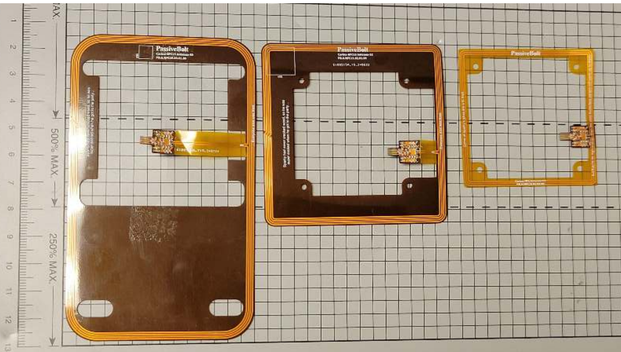
3 NFC ANTENNAS TESTED
